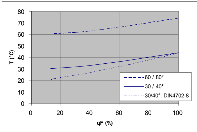
Uitlaatgastemperatuur-diagram van een PYROGAS VARINO in relatie tot de belasting
