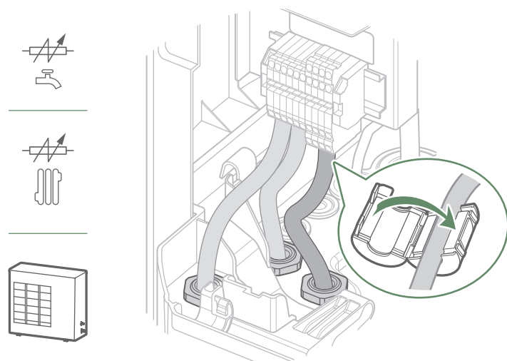
fig. 43 - Passages de câbles
