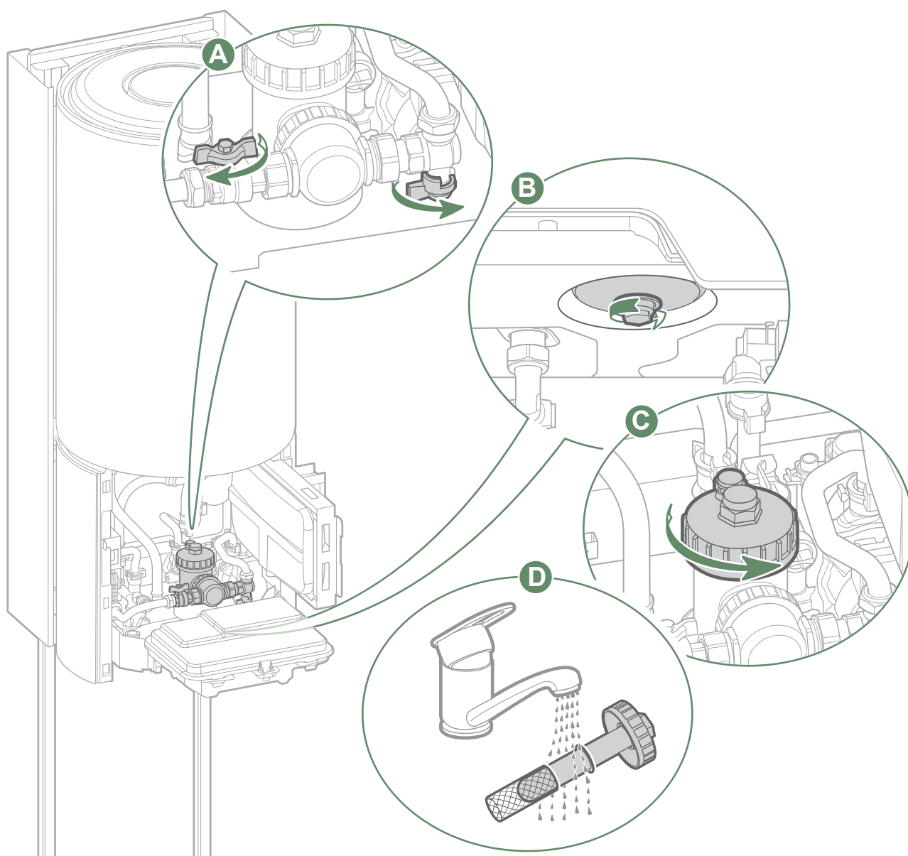
fig. 48 - Nettoyage du pot à boues
