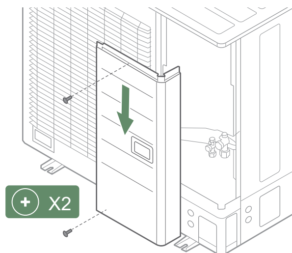
fig. 14 - Ouverture de l'unité extérieur modèle 10
