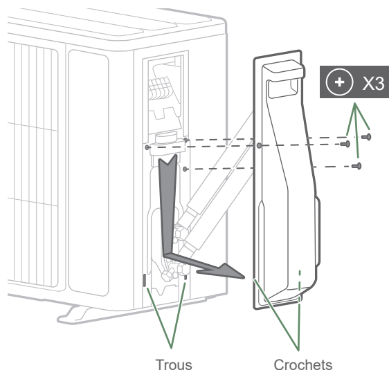
fig. 13 - Ouverture de l'unité extérieur modèles 3/4/6/8
