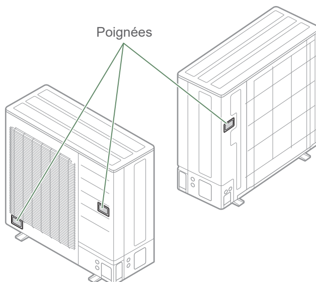
fig. 15 - Transport de l'unité extérieur modèle 10
