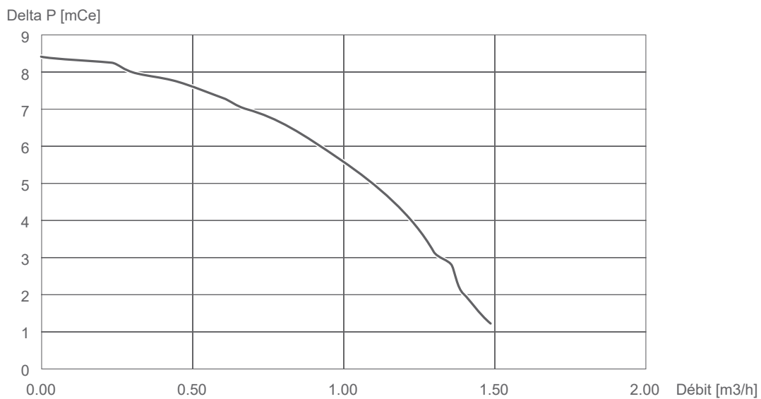
fig. 5 - Vitesse circulateur
