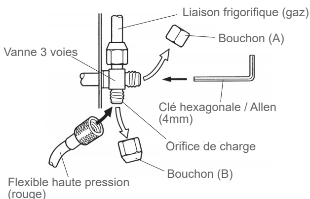
fig. 56 - Raccordement du flexible sur la vanne gaz
