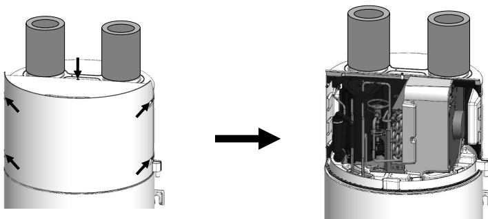
Schroef de voorklep los (x 5 schroeven)
