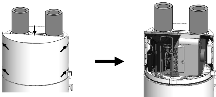
Svitare la copertura anteriore (x 5 viti)
