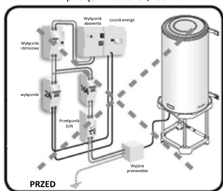
Standardowe podłączenie elektrycznego ogrzewacza wody z przełącznikiem dzień/noc
