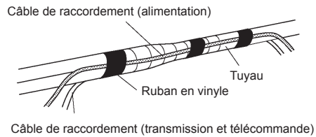
Câble de raccordement (transmission et télécommande)
