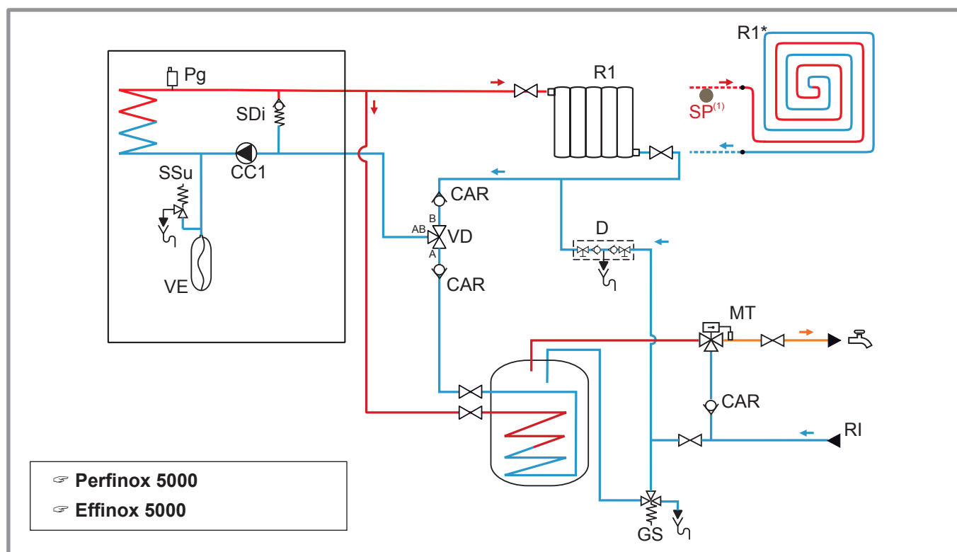
figure 1 - Schéma hydraulique 1 circuit de chauffage direct et ECS
