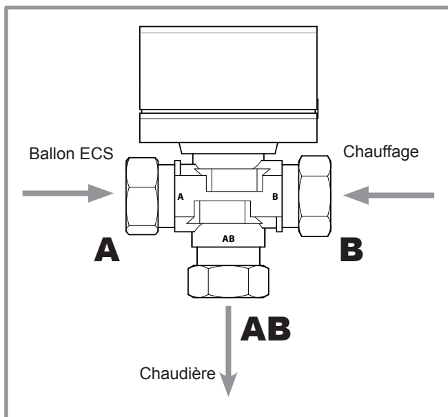
figure 3 - Sens de circulation vanne directionnelle
