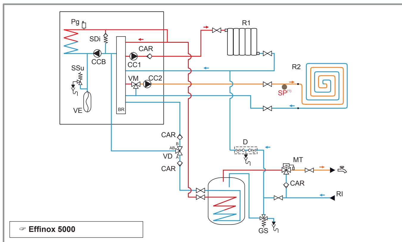
figure 2 - Schéma hydraulique 2 circuits de chauffage (avec kit 2 circuits) et ECS
