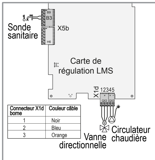
figure 12 - Raccordements électriques (perfinox condens 5000, effinox condens 5000)
