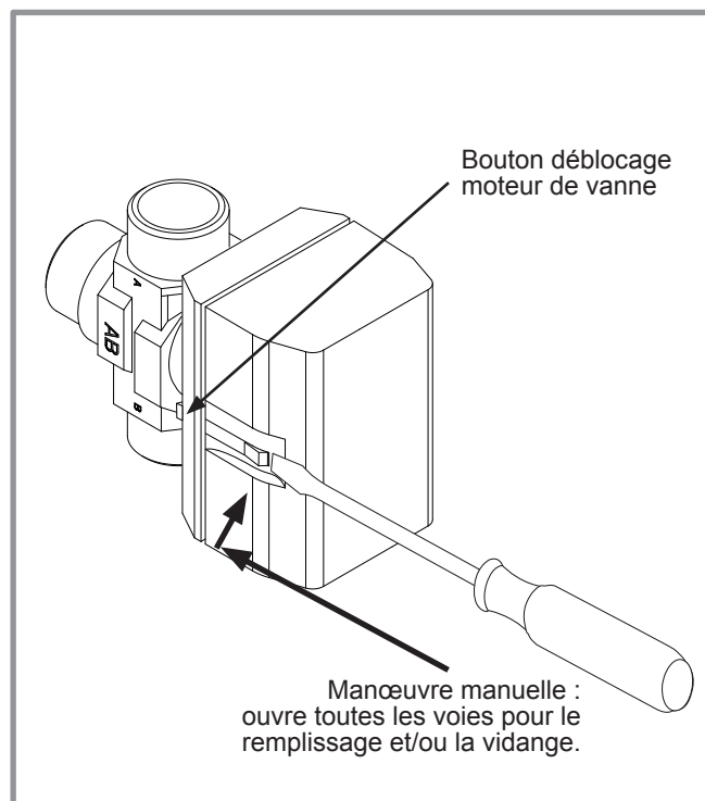
figure 4 - Débrayage - déblocage moteur
