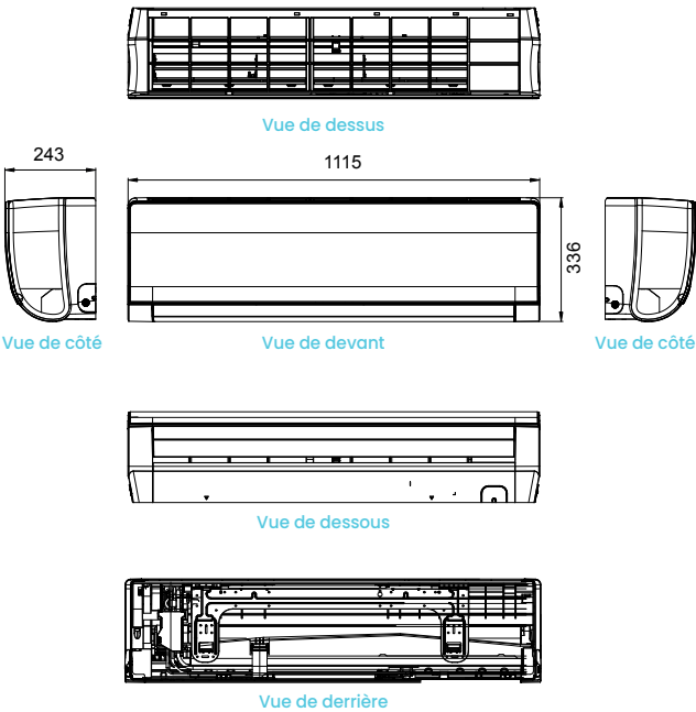
UIM 24 PIB1
