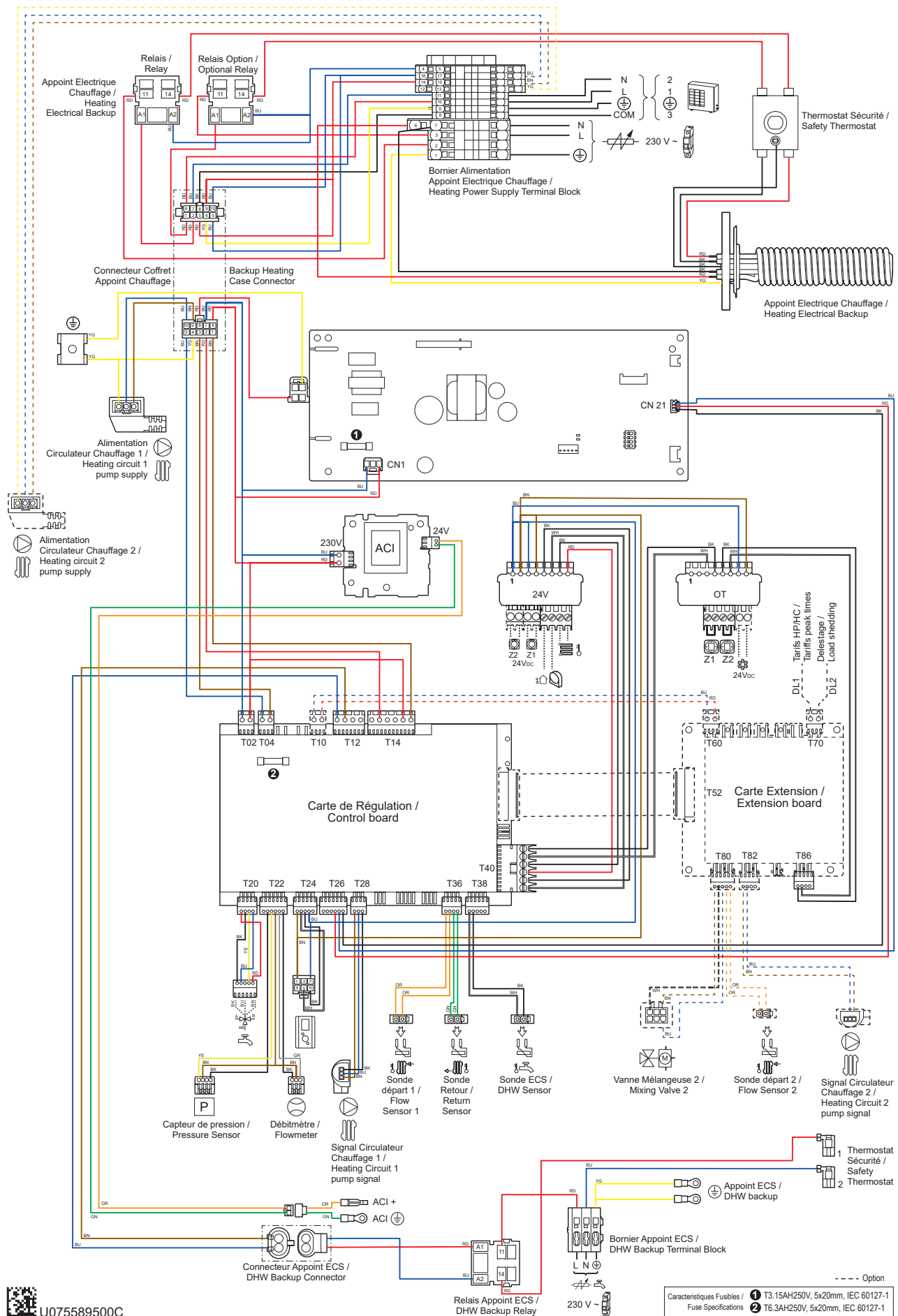
fig. 19 - Câblage électrique Module hydraulique (hors raccordements installateur)
