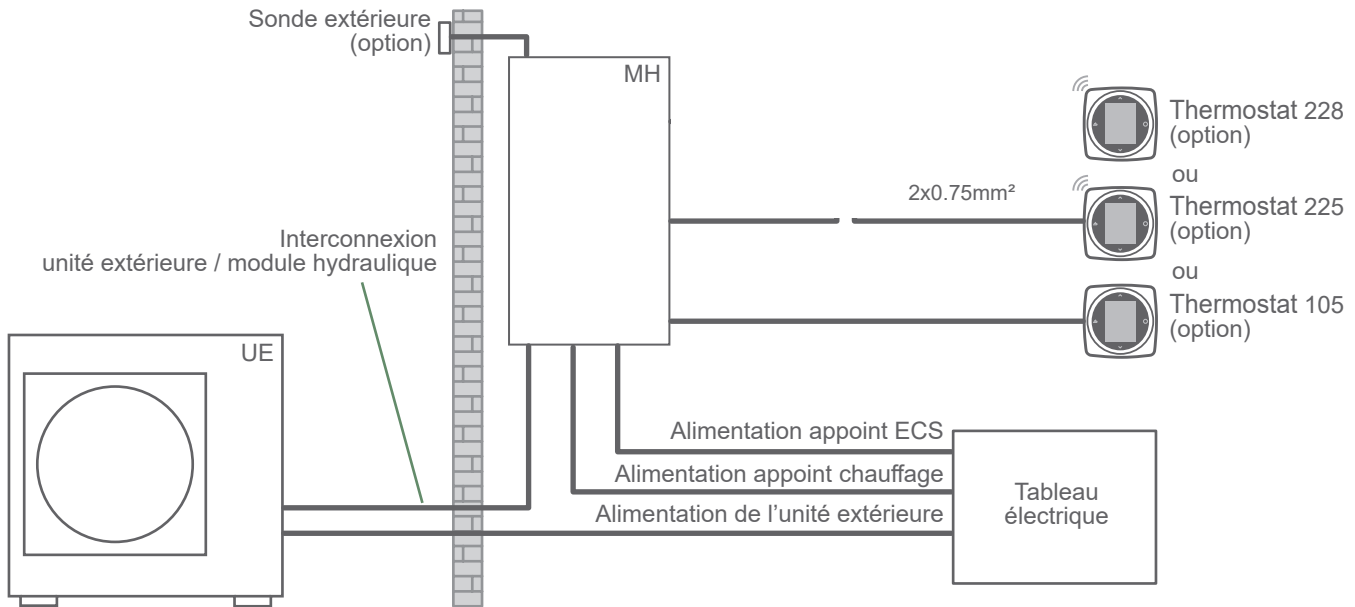
fig. 12 - Schéma d'ensemble des raccordements électriques pour une installation simple (1 circuit de chauffe)
