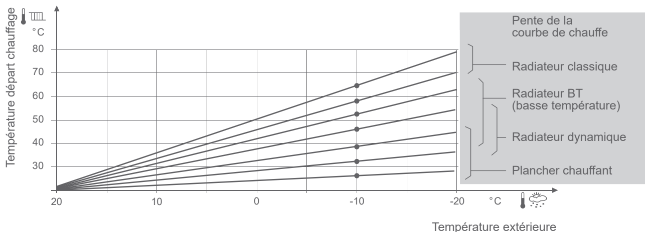
fig. 17 - Pente de la courbe de chauffe
