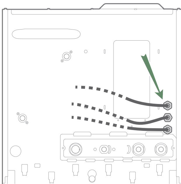
fig. 14 - Passages des câbles
