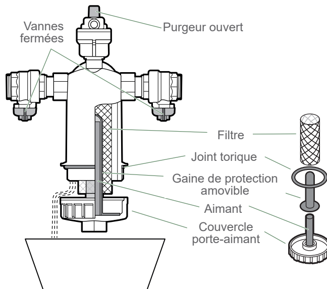
fig. 18 - Nettoyage du pot à boues
