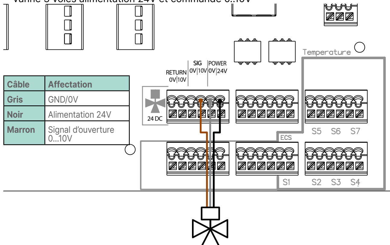
fig. 16 - Raccordement de la vanne 3 voies 0..10V sur RUBIS EVO
