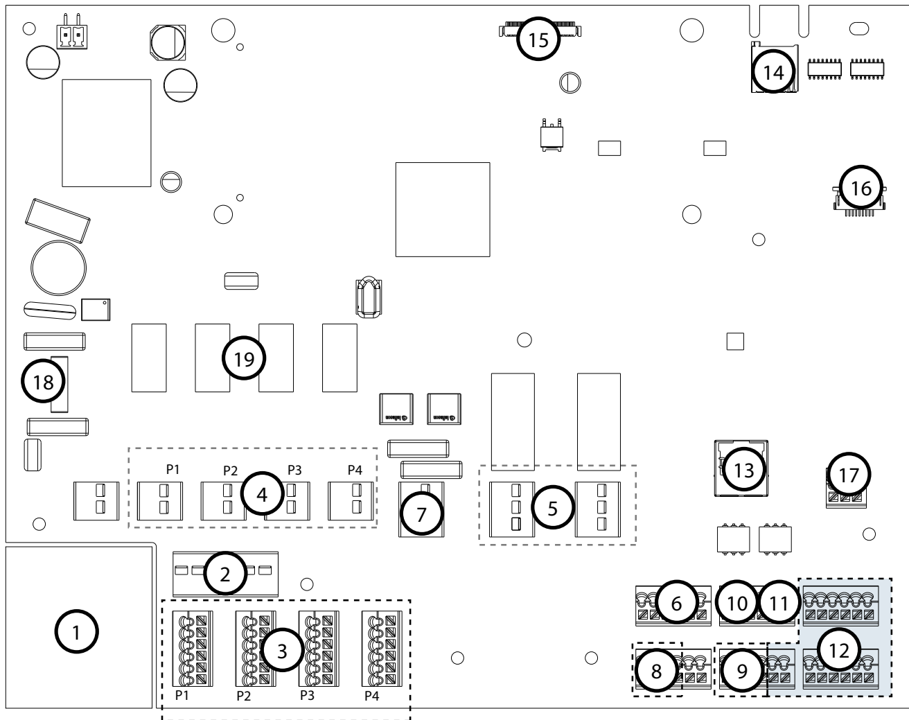
fig. 15 - Raccordements électriques RUBIS EVO
