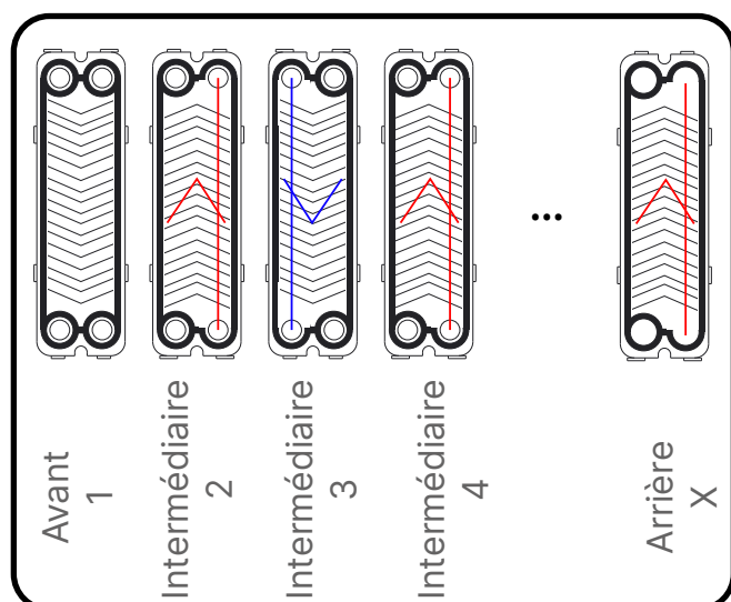
fig. 21 - Empilement de plaques parallèles
