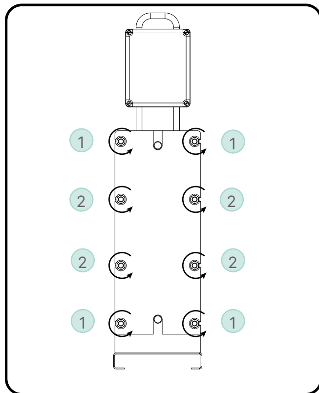
fig. 20 - Échangeur à plaque
