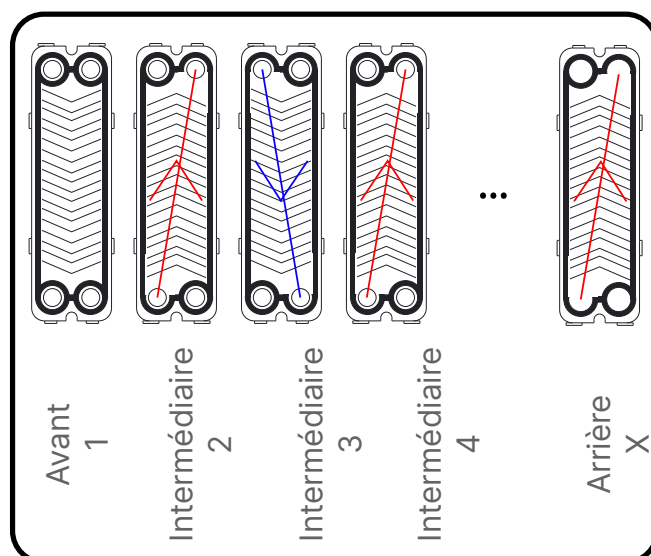
fig. 22 - Empilement de plaques diagonales
