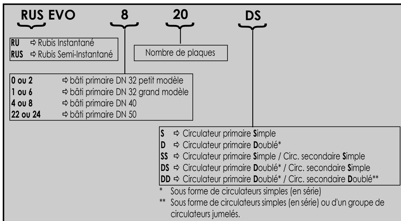
fig. 1 - Plaque signalétique
