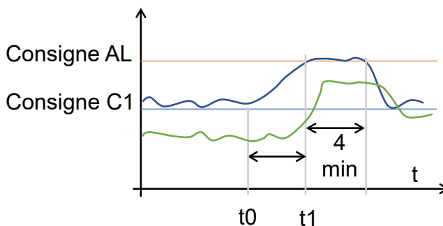
fig. 19 - Température de sonde surveillée
