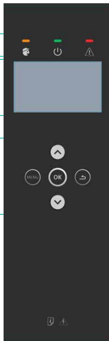
fig. 18 - Interface utilisateur
