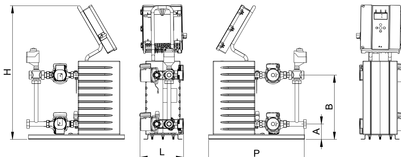
fig. 3 - Dimensions en mm (représentation RUBIS EVO Semi-Instantané)
