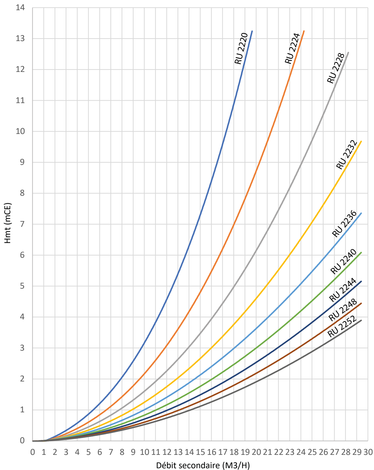
fig. 29 - Pertes de charge gamme 2000
