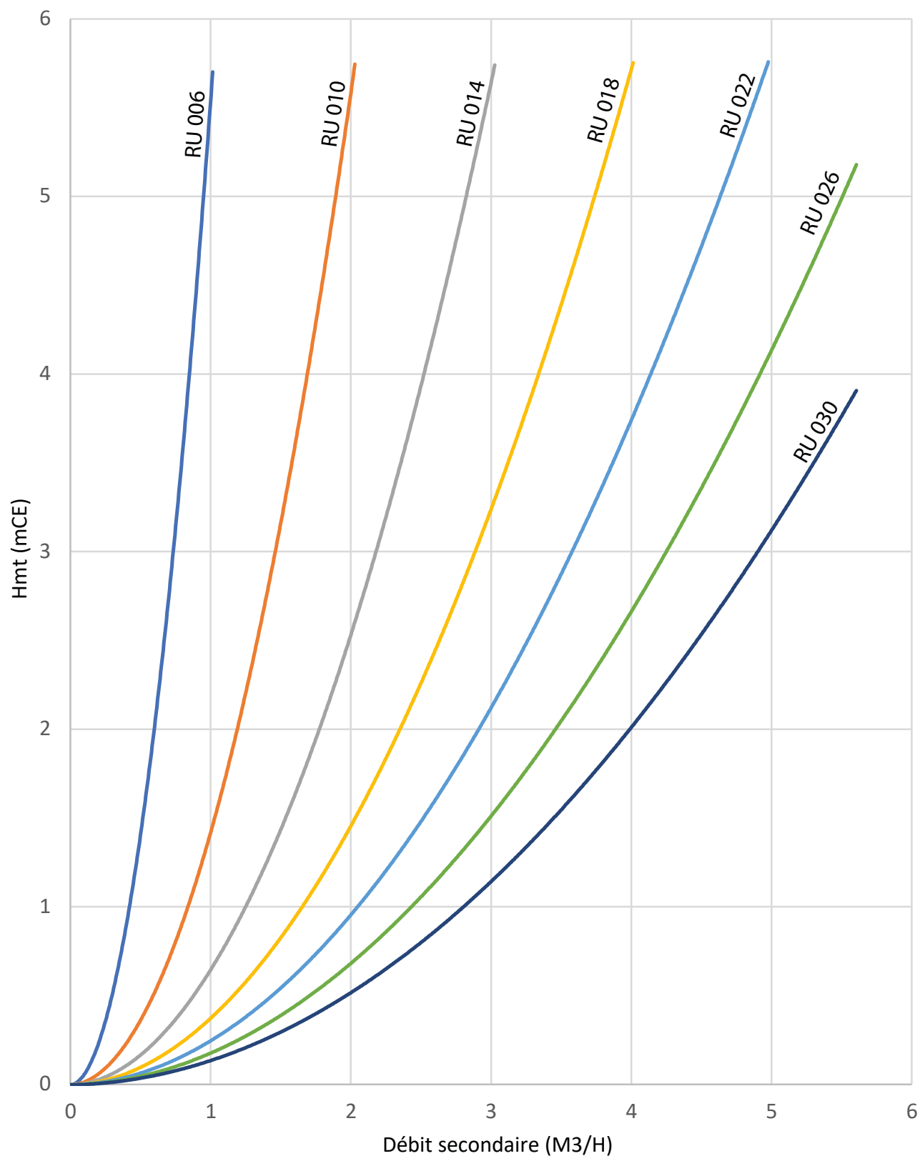
fig. 26 - Pertes de charge gamme 000
