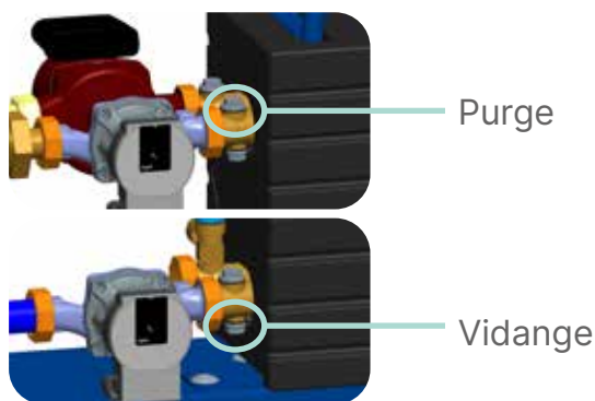
fig. 6 - Position des purges et vidanges sur les RUBIS EVO 000/100/200/600
