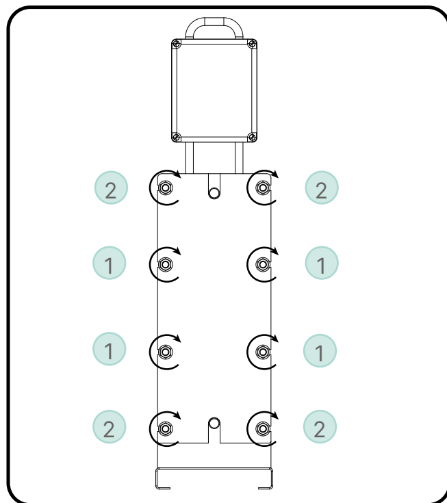
fig. 25 - Fermeture échangeur
