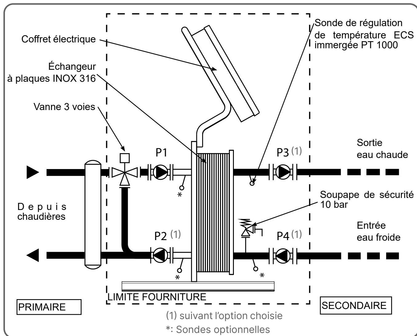
fig. 2 - RUBIS EVO semi instantané
