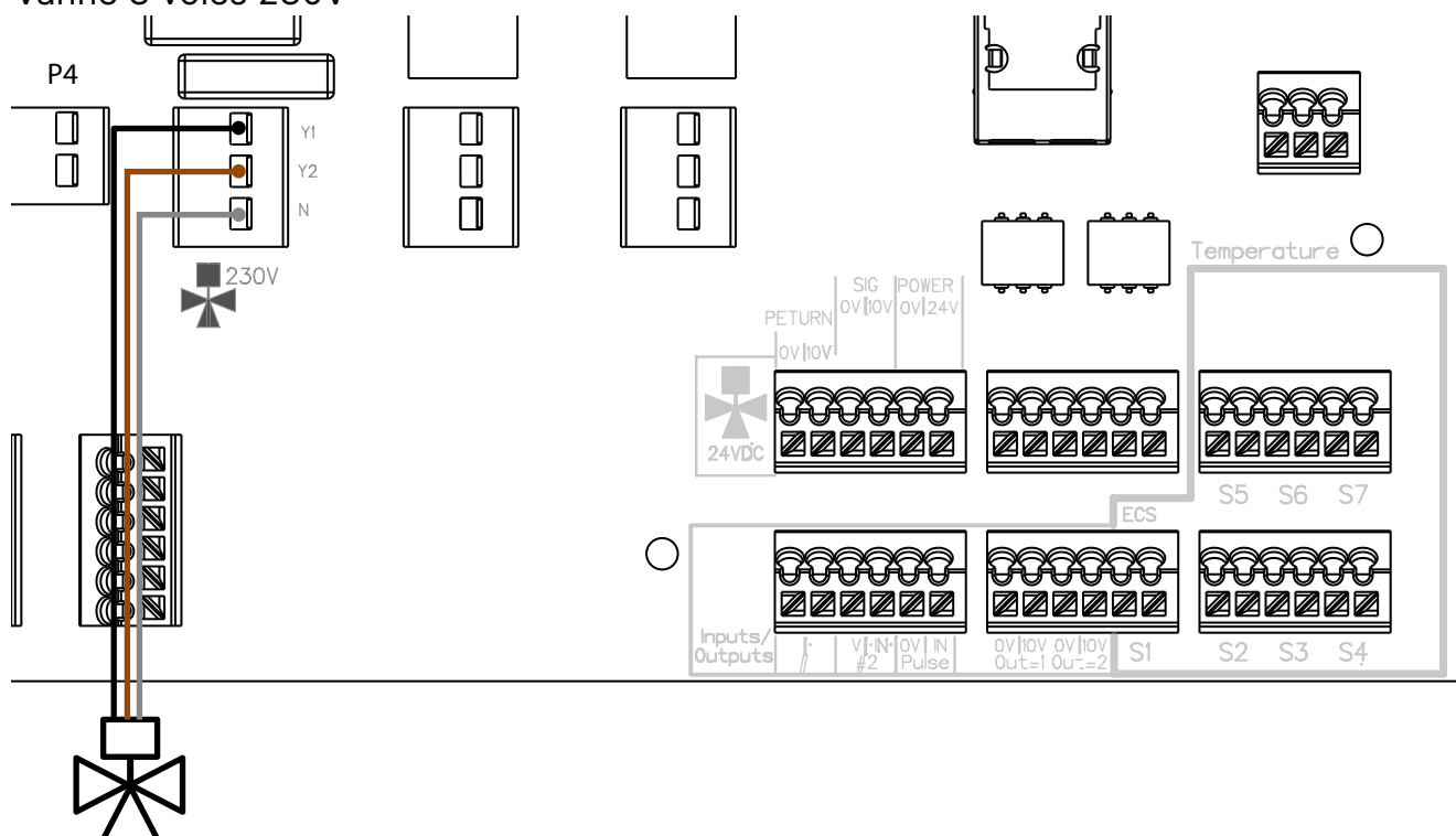
fig. 17 - Raccordement d'une vanne 3 voies 230V (ancienne génération de Rubis, Duplex...)
