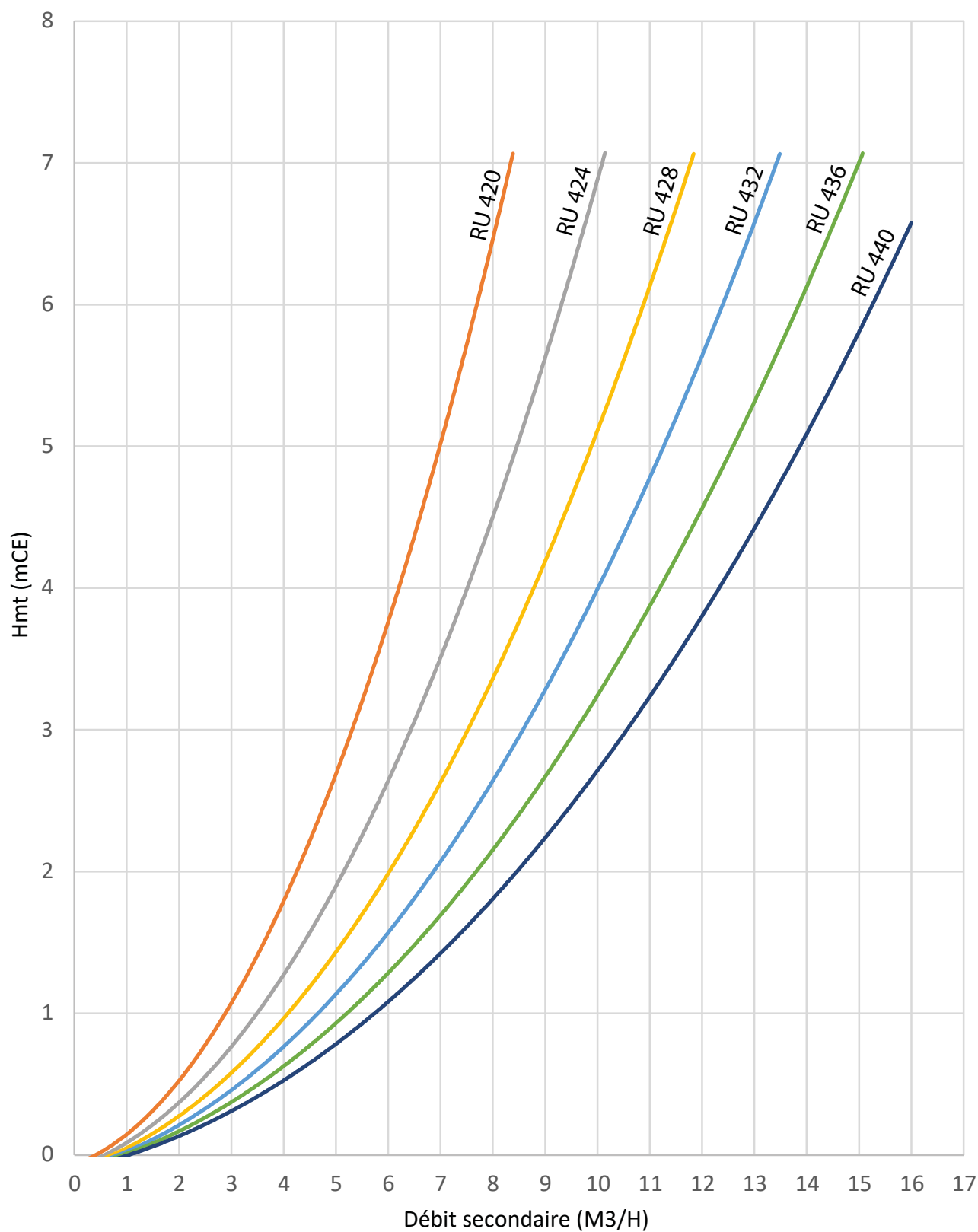
fig. 28 - Pertes de charge gammes 400
