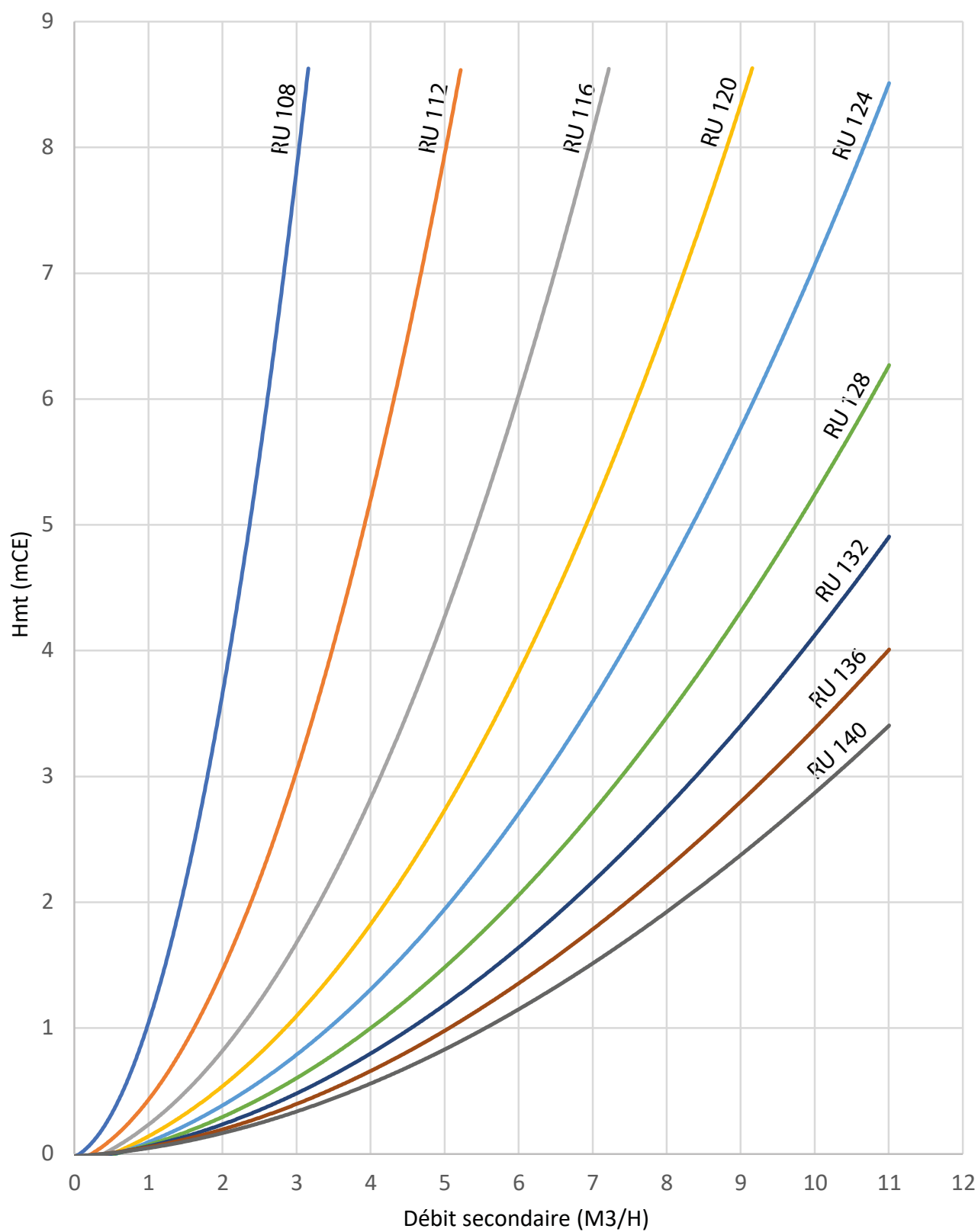
fig. 27 - Pertes de charge gammes 100
