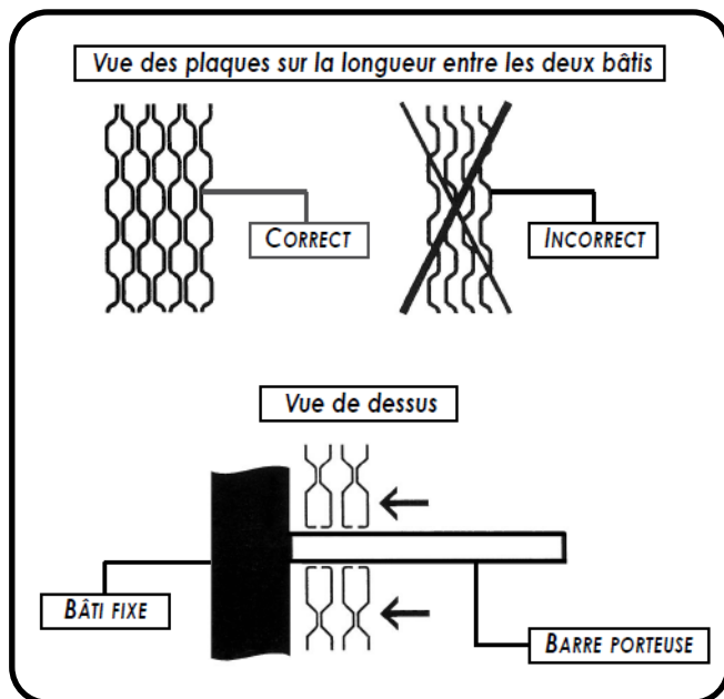
fig. 23 - Position des plaques
