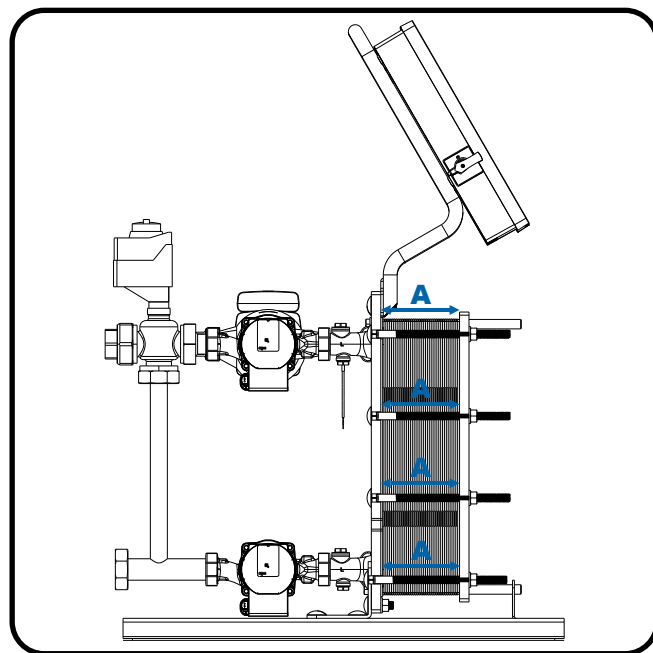
fig. 24 - Vue échangeur sur longueur
