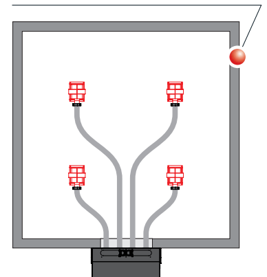
Lagerraum quadratisch
