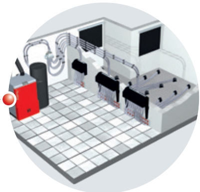
Système d'aspiration triple des granulés RS 4 / RS 8
