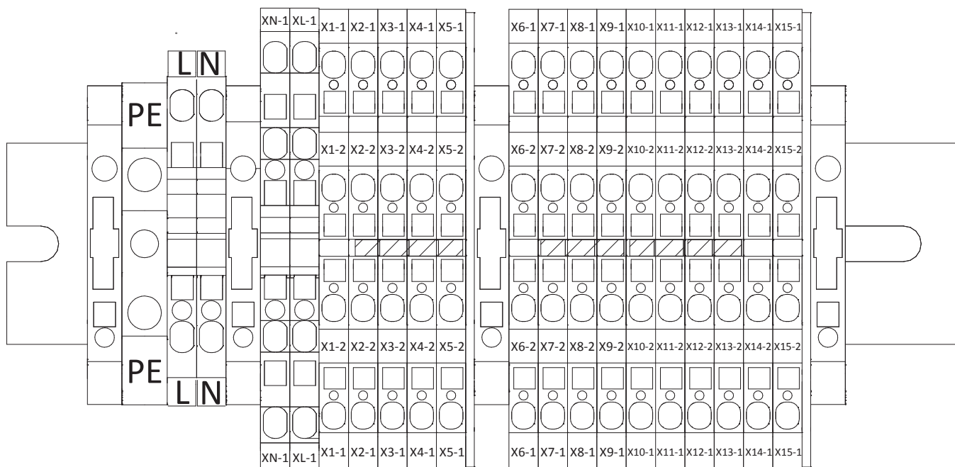
Bloque de terminales del módulo externo:
