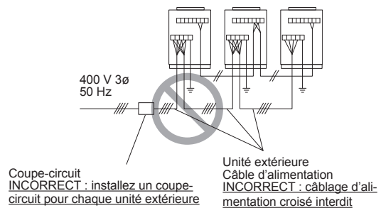
(3) Exemple de mauvais câblage du coupe-circuit
