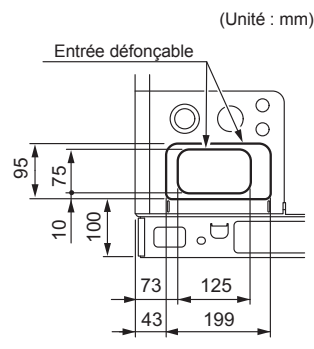
Fig.C Détail de la position de l'entrée défonçable (avant)
