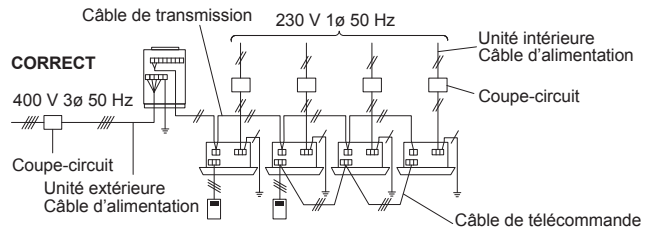
Fig. Si une unité extérieure est raccordée
