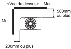
Lorsque l'installation s'effectue avec l'AVANT de l'unité extérieure face au mur Fig. 10
