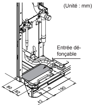
Fig.B Détail de la position de l'entrée défonçable (bas)
