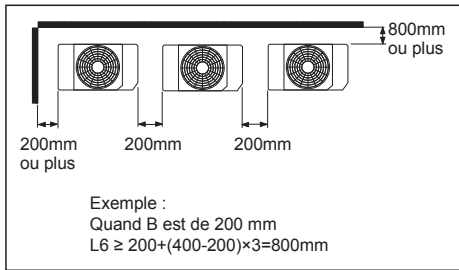
Lorsque l'installation s'effectue avec l'AVANT de l'unité extérieure face au mur Fig. 10
