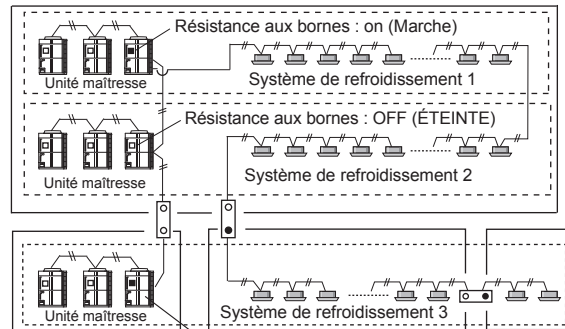
Figure : Réglage de la résistance aux bornes
