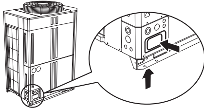
Fig.B Détail de la position de l'entrée défonçable (bas)
