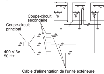
(3) Exemple de mauvais câblage du coupe-circuit
