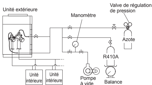
Fig. A Système de raccordement
