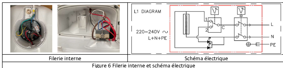
Figure 6 Filerie interne et schéma électrique
