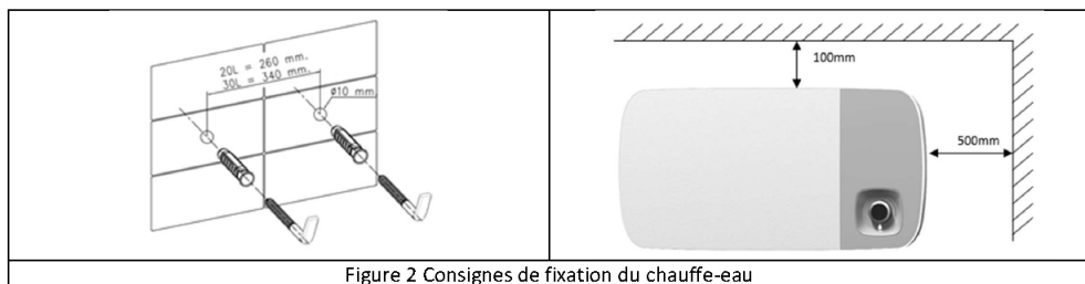
Figure 2 Consignes de fixation du chauffe-eau
