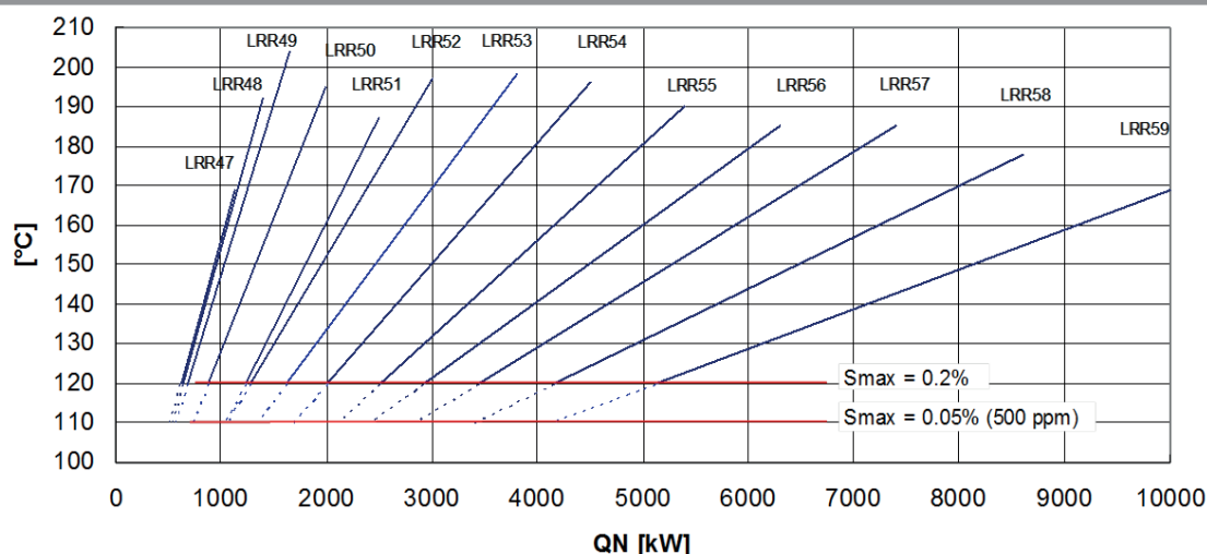
figura 7 - Temperatura dei fumi LRR, gasolio con caldaia pulita
