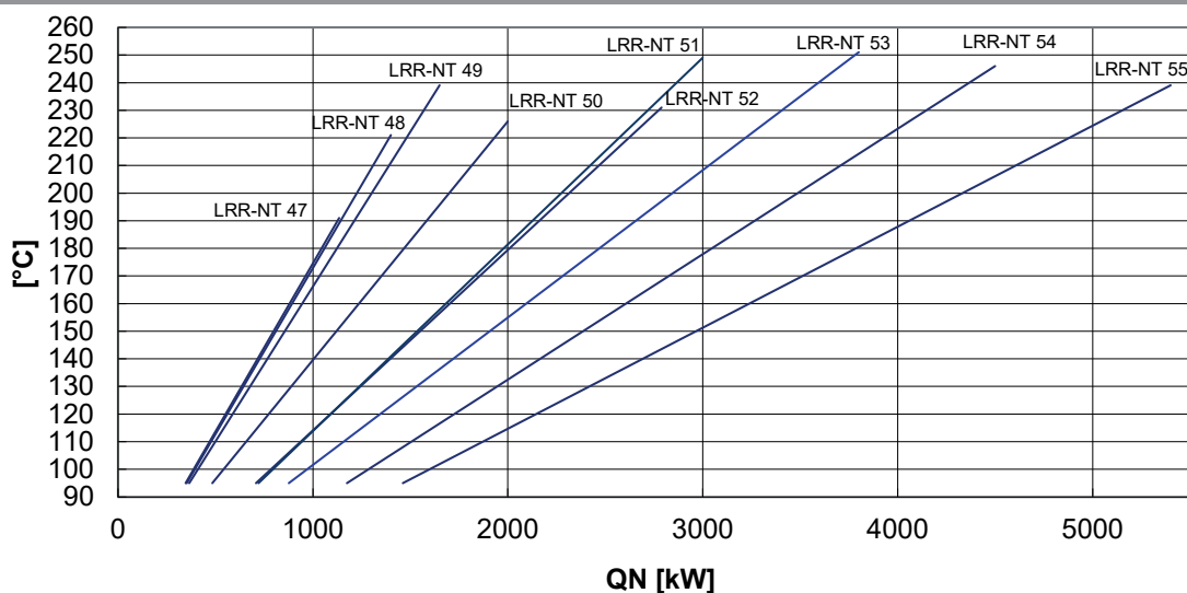
figura 10 - Temperatura dei fumi LRR-NT, metano con caldaia pulita
