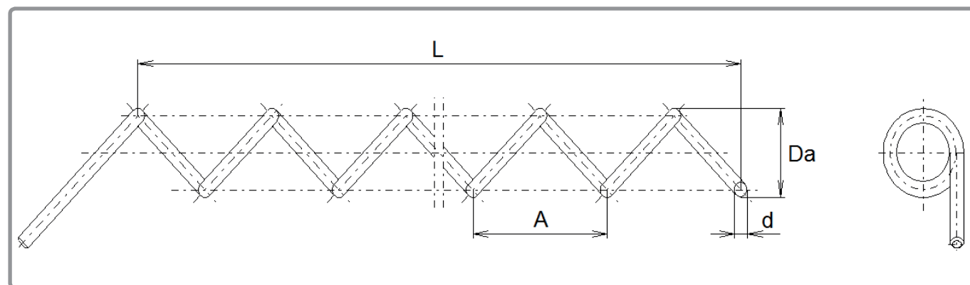
figura 15 - Turbulatori
