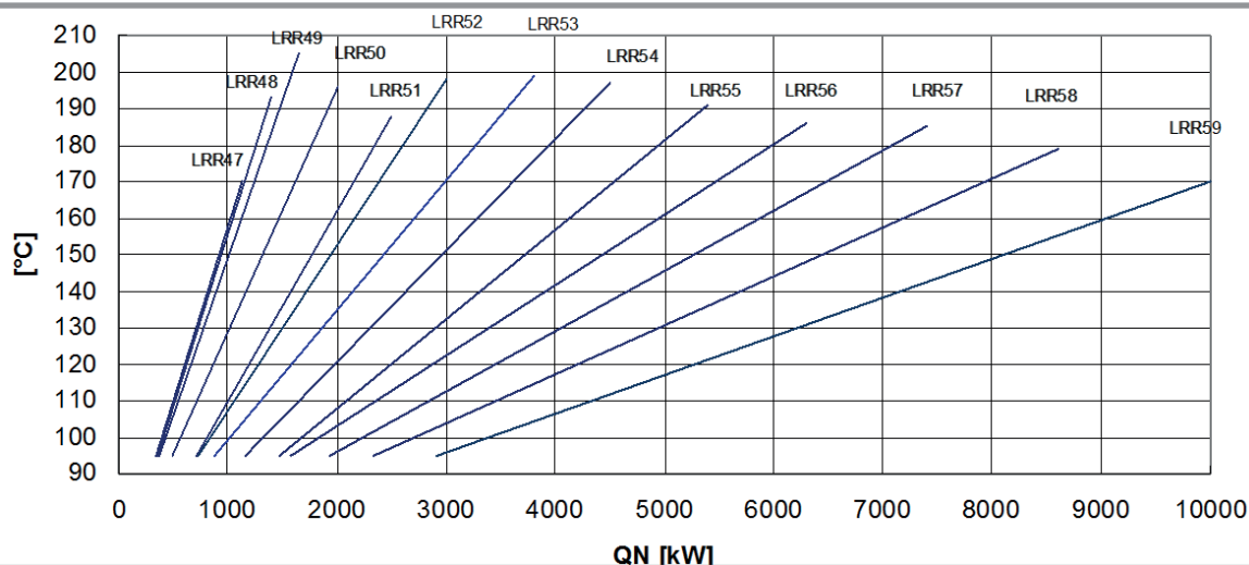
figura 8 - Temperatura dei fumi LRR, metano con caldaia pulita
