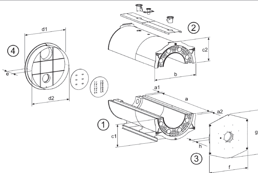
figura 6 - Dimensioni versione sezionata
