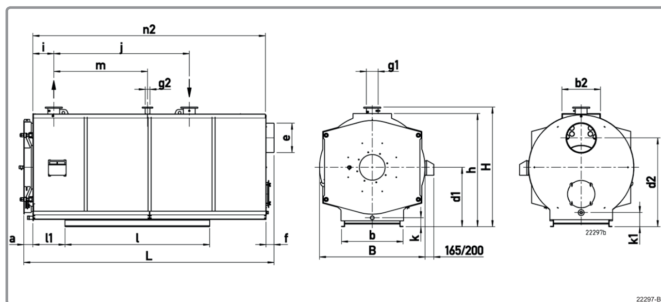
figura 3 - LRR / LRR-NT 53-59
