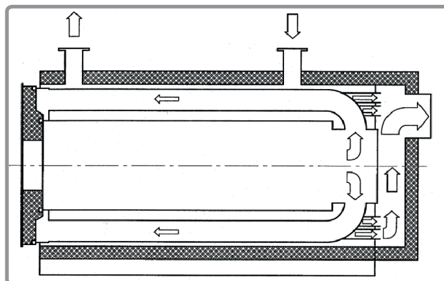
figura 1 - 3 tiraggi
