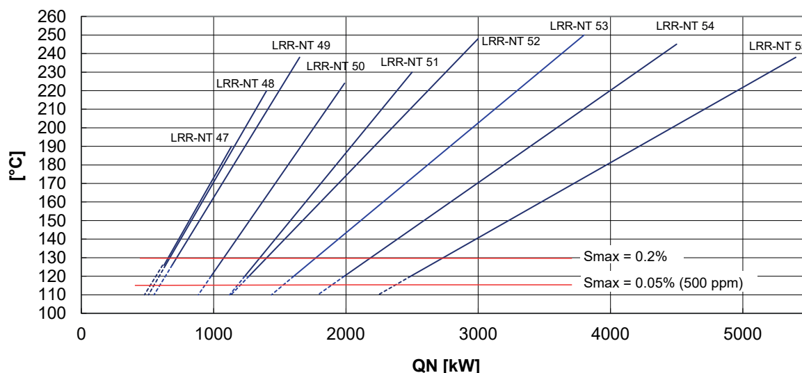
figura 9 - Temperatura dei fumi LRR-NT, gasolio con caldaia pulita
