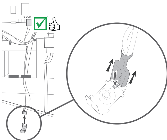
fig. 40 - Perfinox 2 Duo - Débrancher le câble de terre
