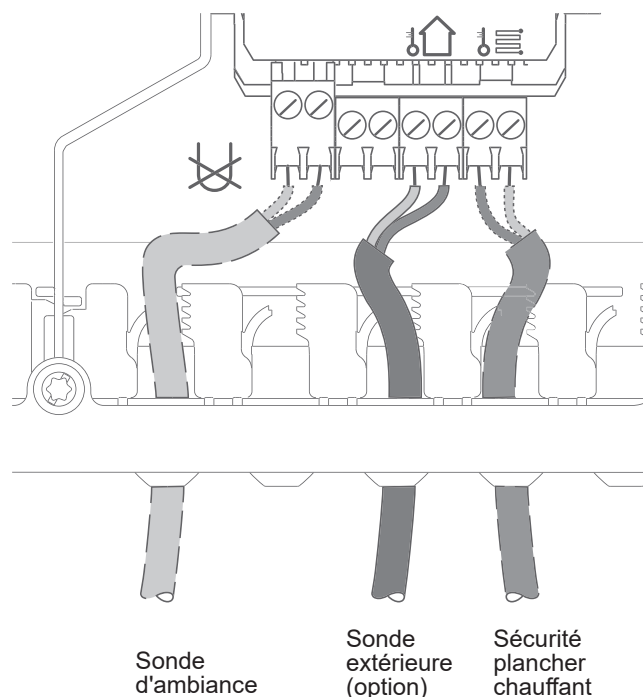
fig. 25 - Accès borniers TBTS
