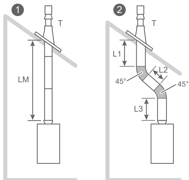
Raccordement ventouse type C33
