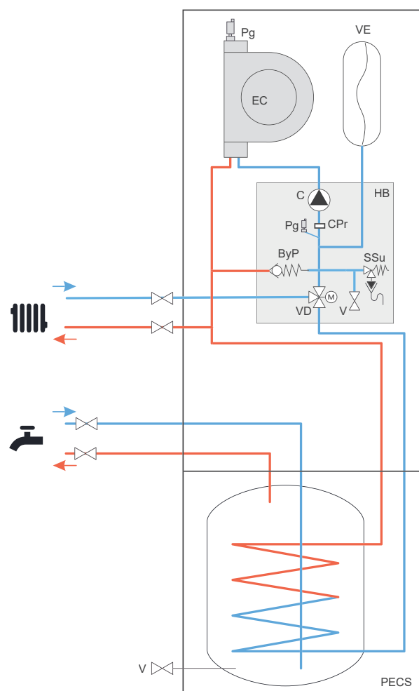
fig. 7 - Principe hydraulique
