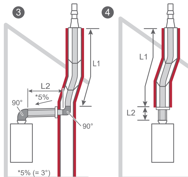
Raccordement ventouse type C93
