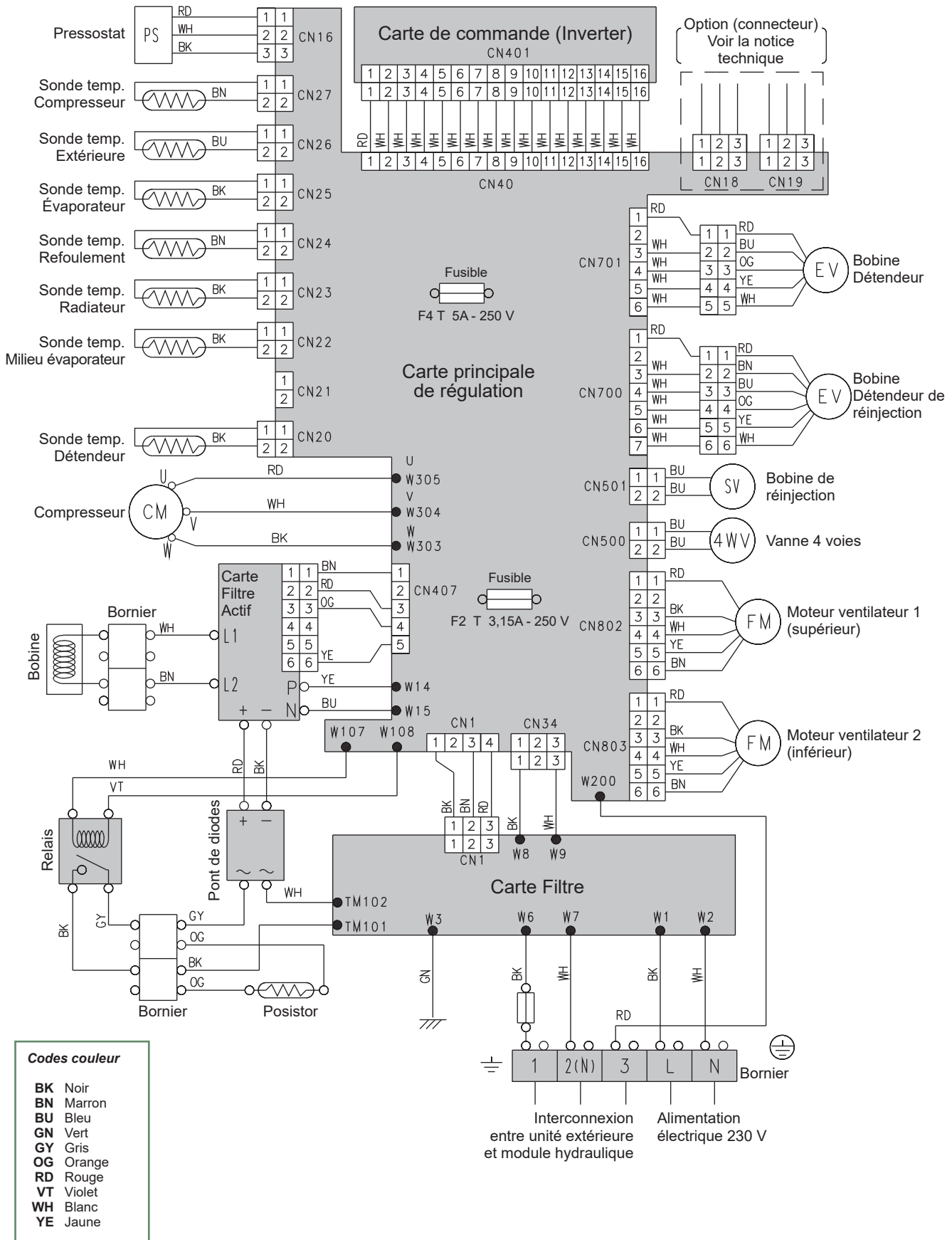
fig. 55 - Câblage électrique unité extérieure modèle monphasée
