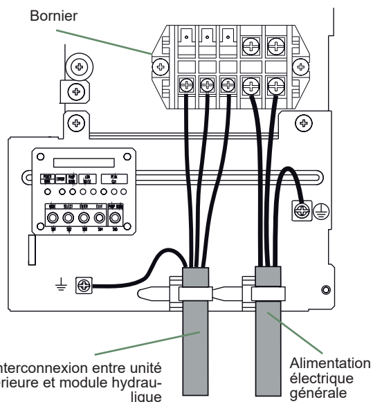
fig. 39 - Connexions au bornier de l'unité extérieure monophasée
