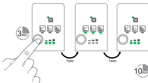
fig. 32 - Mode dégazage
