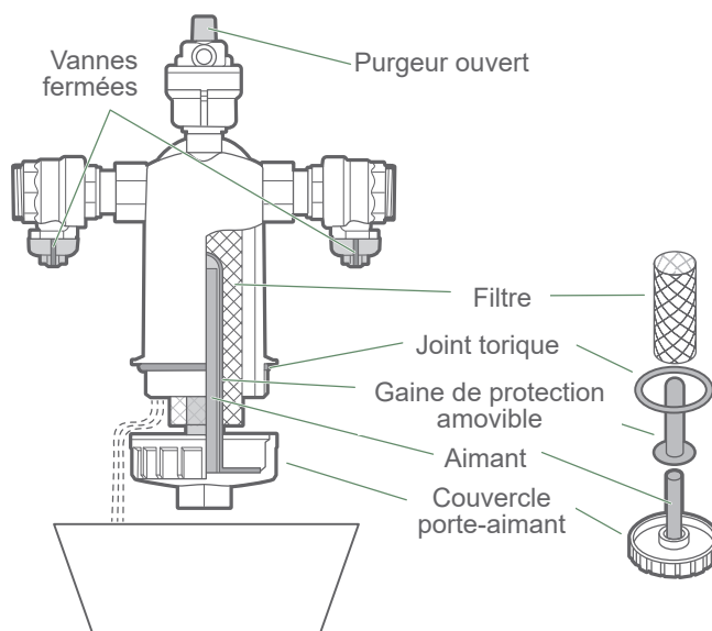
fig. 12 - Nettoyage du pot à boues
