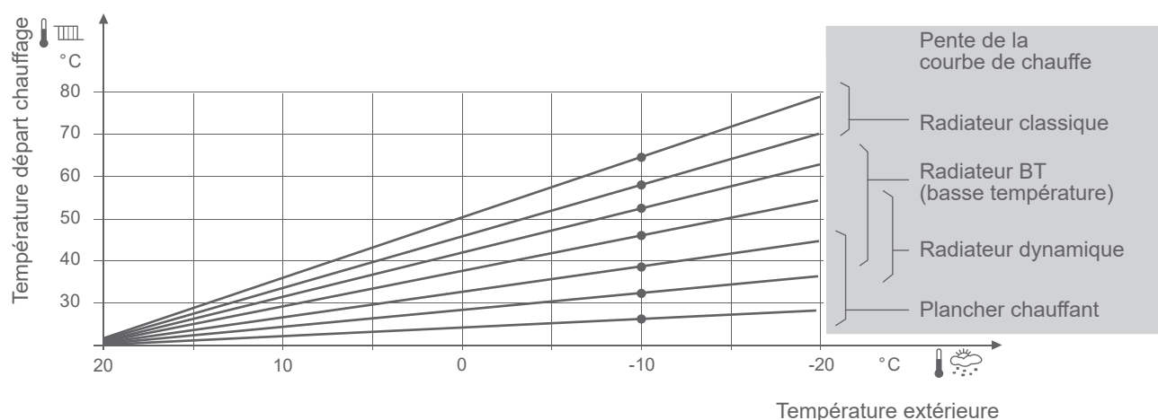
fig. 11 - Pente de la courbe de chauffe
