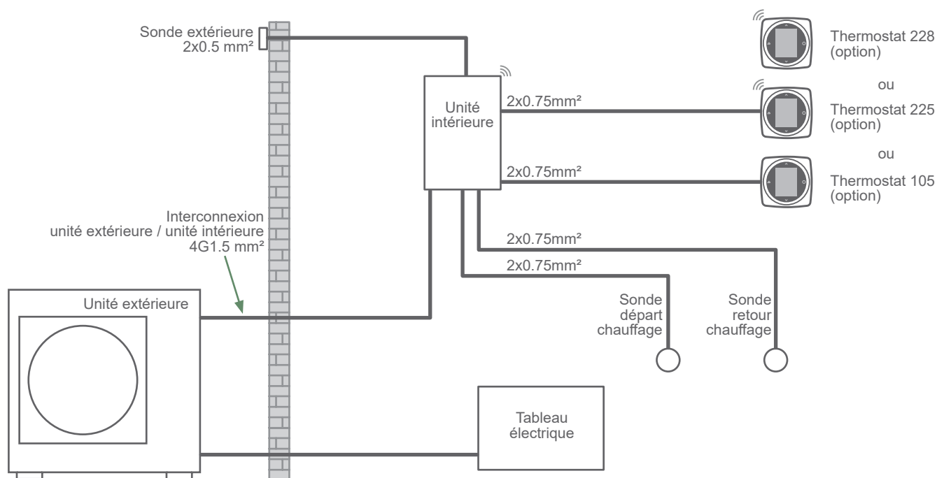
fig. 7 - Schéma d'ensemble des raccordements électriques pour une installation simple (1 circuit de chauffe)
