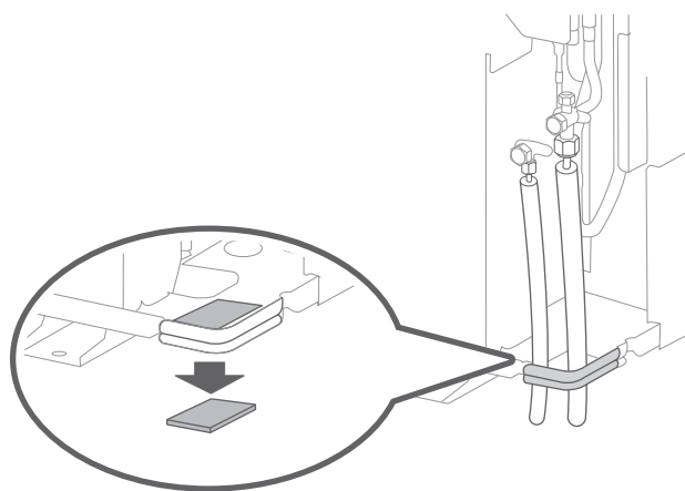
■ Connexion par le bas
