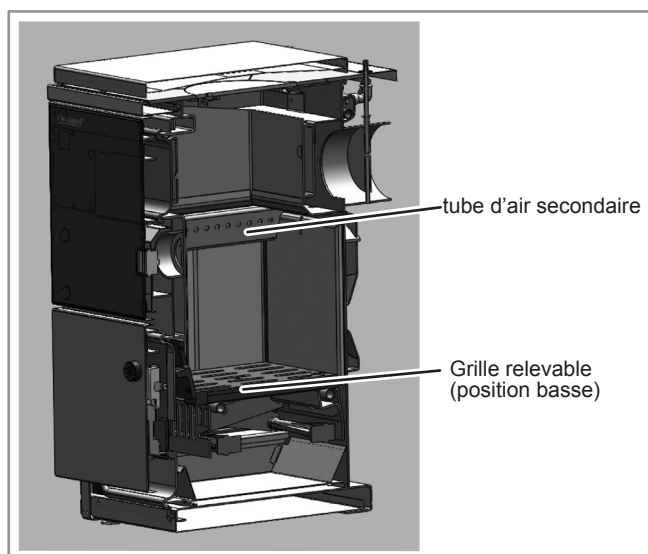
fig. 23 - Grille relevable (position basse) : espace de remplissage maximal
