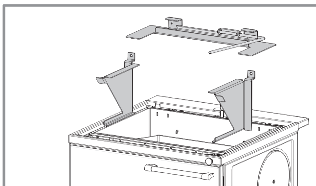
fig. 26 - Dépose des tôles déflectrices
