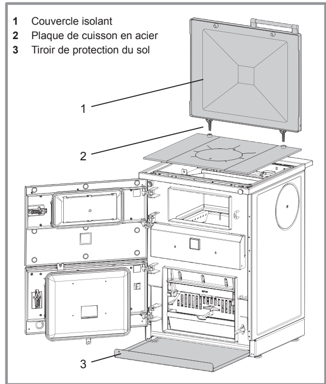
fig. 7 - Installation de la plaque de cuisson en acier, du couvercle isolant et du tiroir de protection du sol
