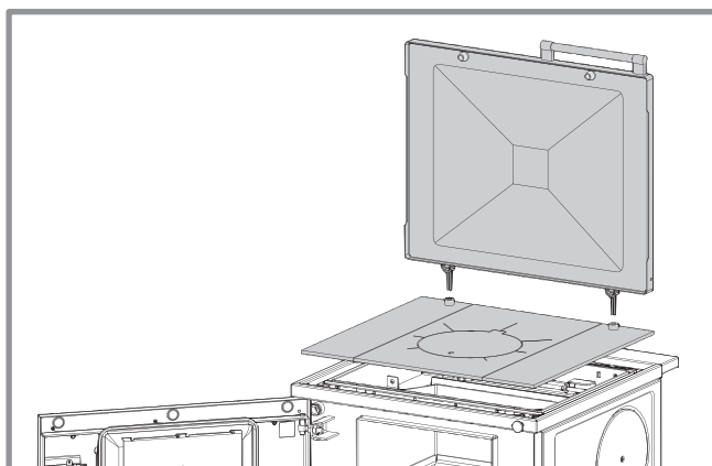
fig. 25 - Dépose couvercle isolant et plaque de cuisson
