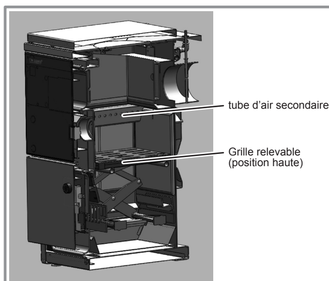
fig. 24 - Grille relevable (position haute) : espace de remplissage réduit
