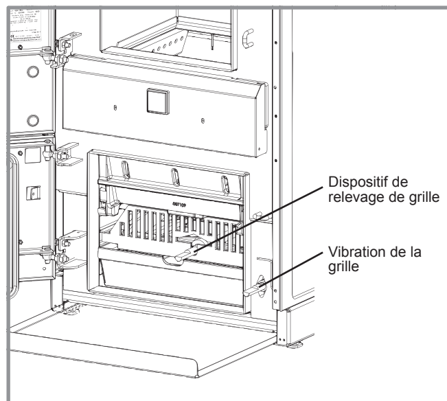
fig. 27 - Graissage de l'agitateur et du dispositif de relevage de grille
