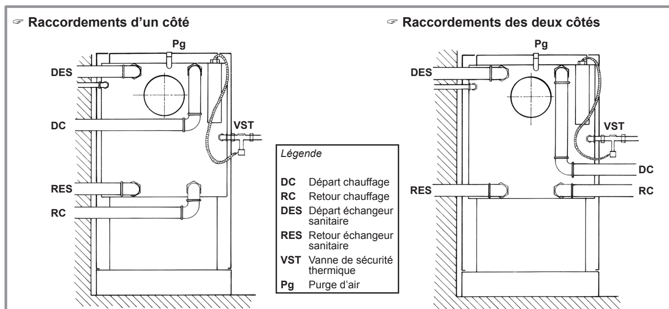
fig. 13 - Raccordements et vanne de sécurité thermique
