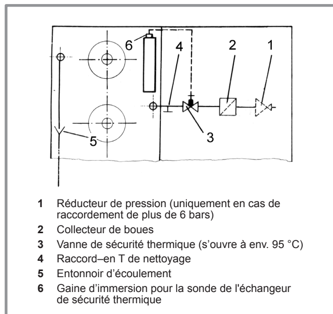
fig. 14 - Raccordement de l'échangeur de sécurité thermique
