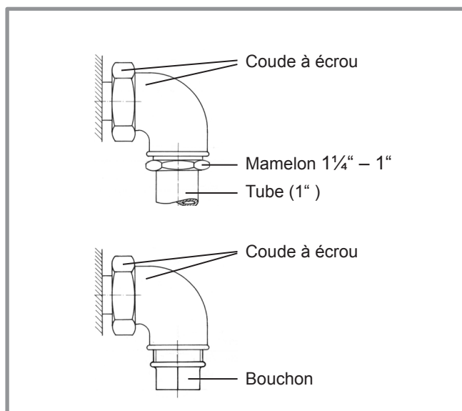
fig. 12 - Mise en place des coudes à écrou
