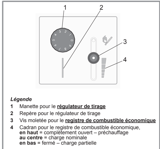
fig. 17 - Régulateur de tirage et registre de combustible économique
