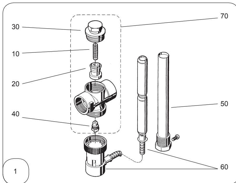
fig. 32 - Vanne de sécurité thermique – accessoires
