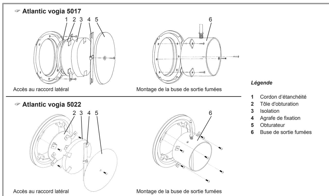
fig. 9 - Suppression de l'obturateur et montage de la buse de sortie fumées
