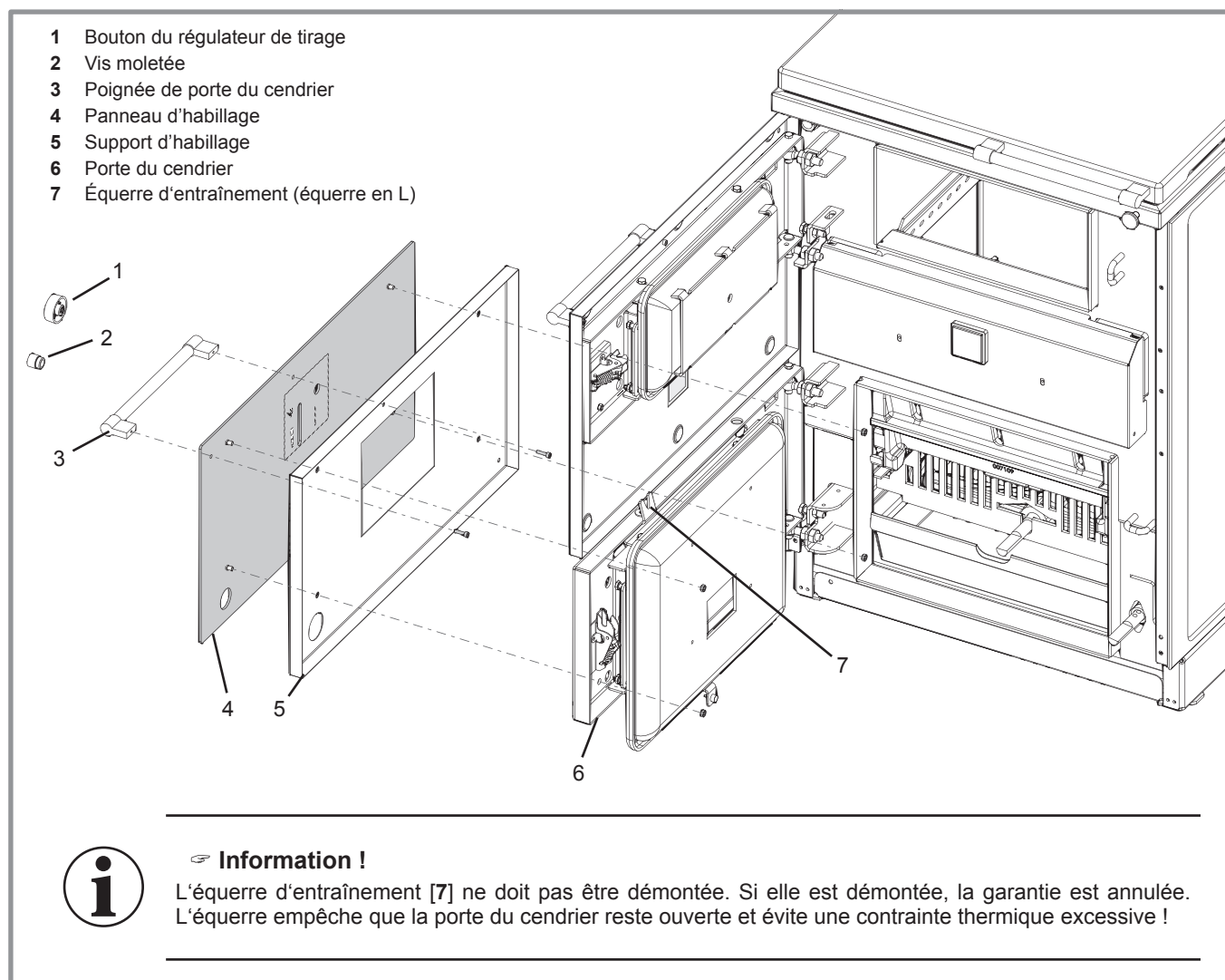
fig. 8 - Montage du panneau de protection décoratif
