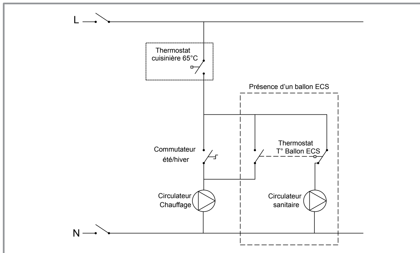
fig. 15 - Schéma électrique de principe
