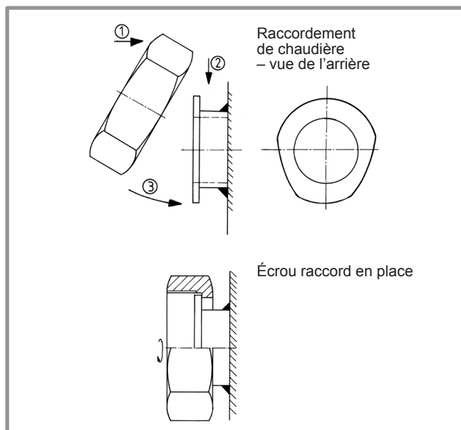
fig. 11 - Mise en place de l'écrou raccord
