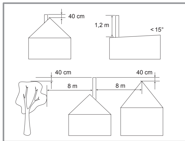
fig. 10 - Hauteur de la souche du conduit d'évacuation
