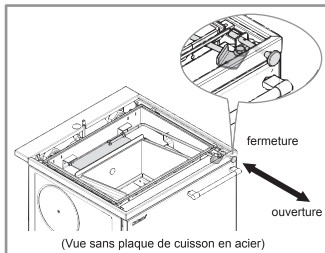
fig. 19 - Ouverture / Fermeture du clapet de préchauffage
