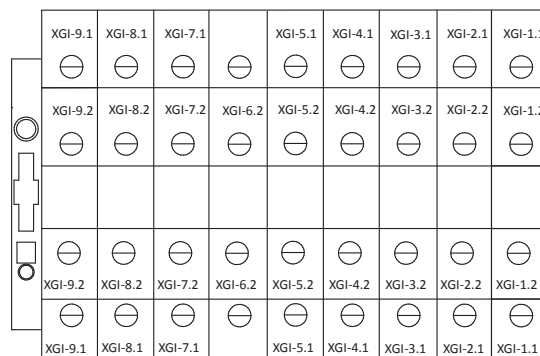
Morsettiera GI
