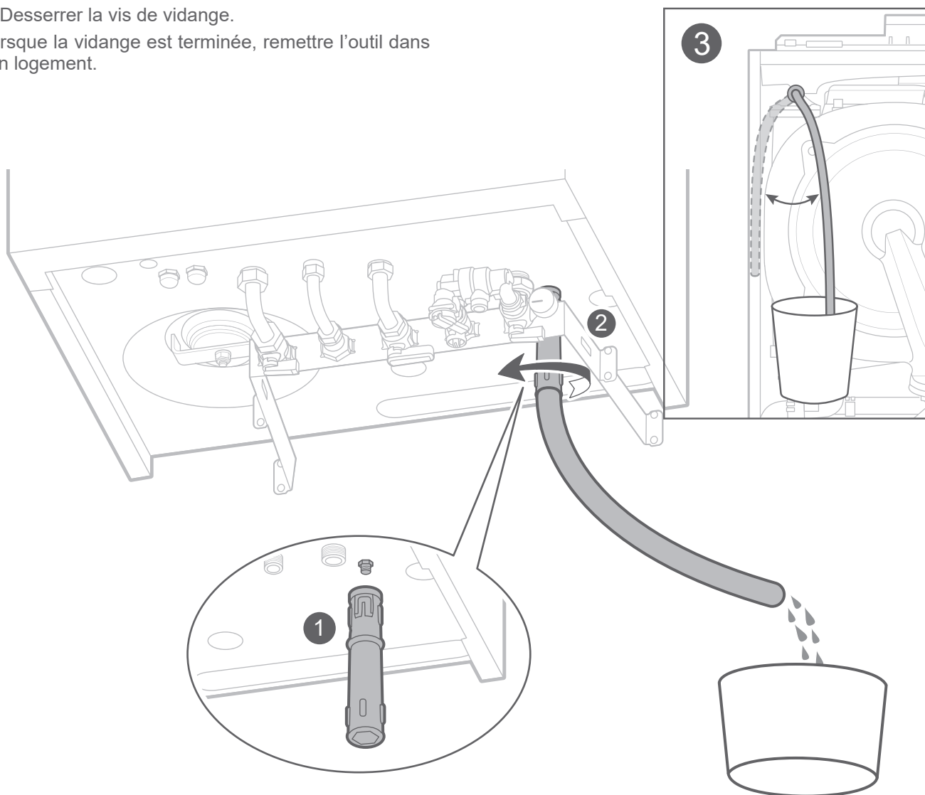
fig. 26 - Vidange de la chaudière
