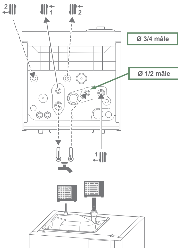
fig. 2 - Repérage hydraulique
