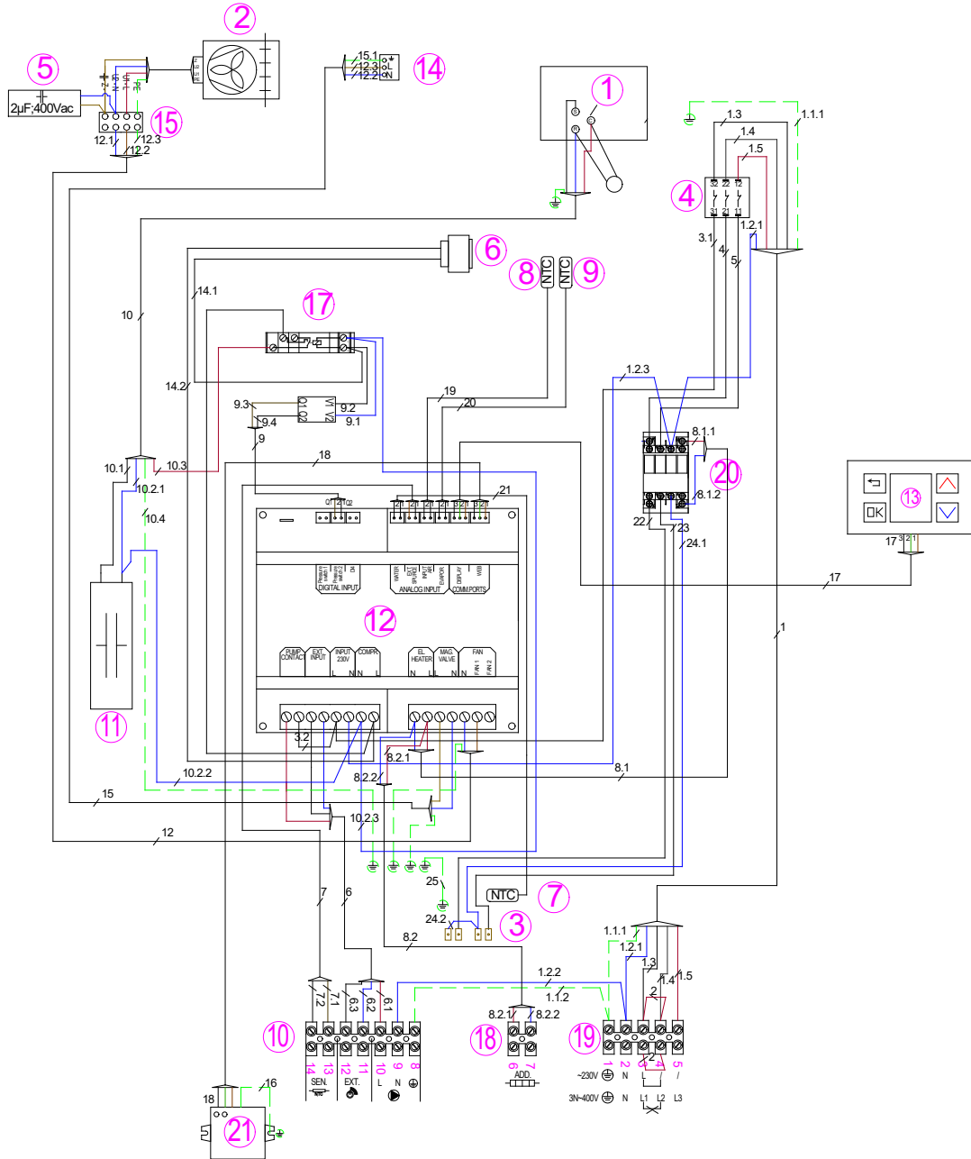
Figure 8: Schéma électrique
