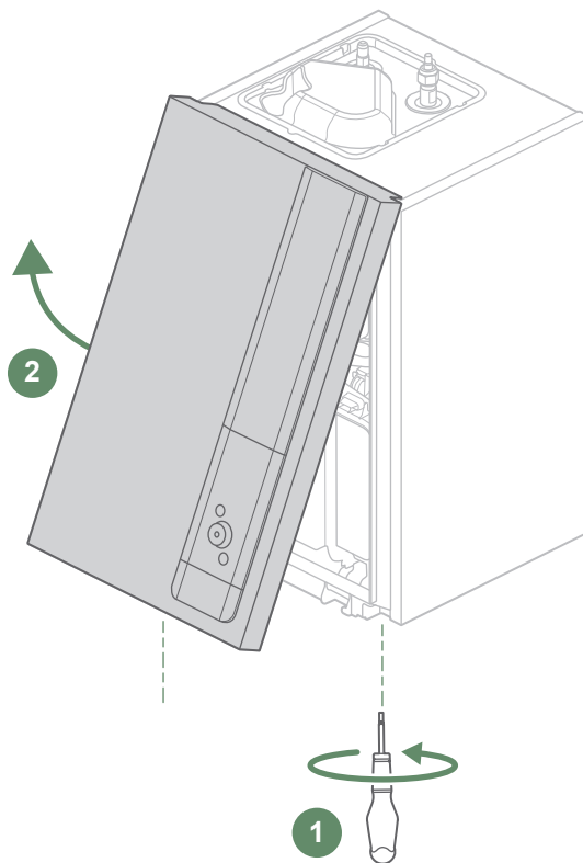
fig. 21 - Ouverture de la façade
