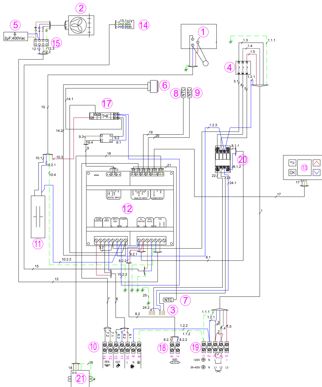
Figure 8: Schéma électrique
