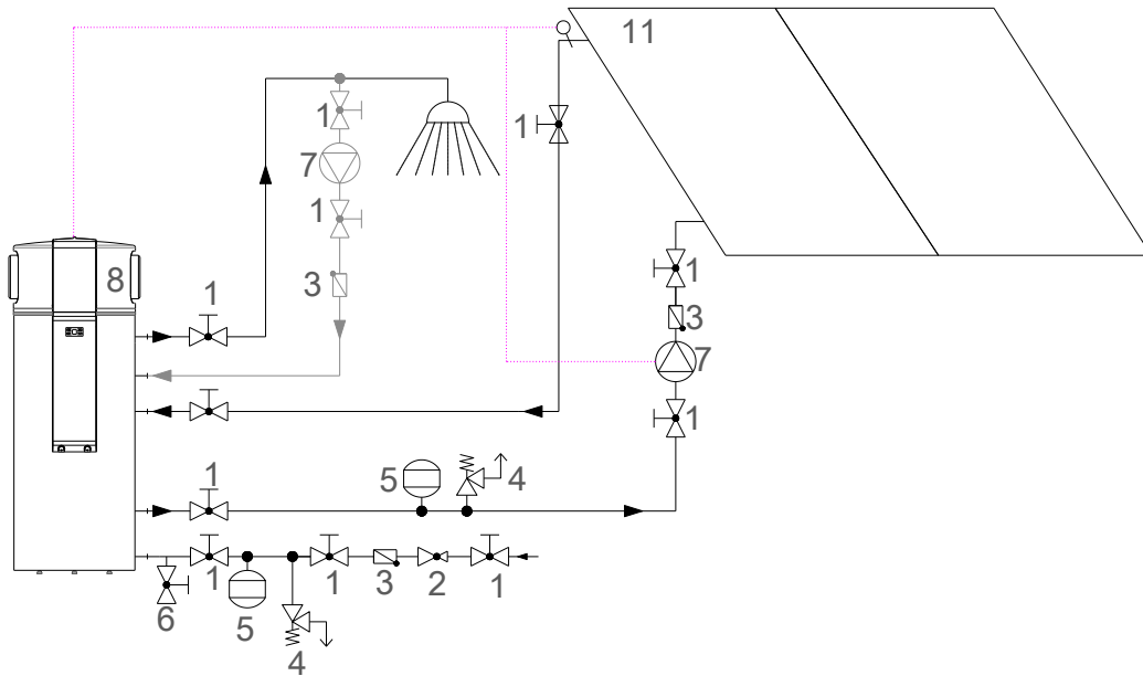
Figure 4: Pompe à chaleur combinée à des capteurs solaires
