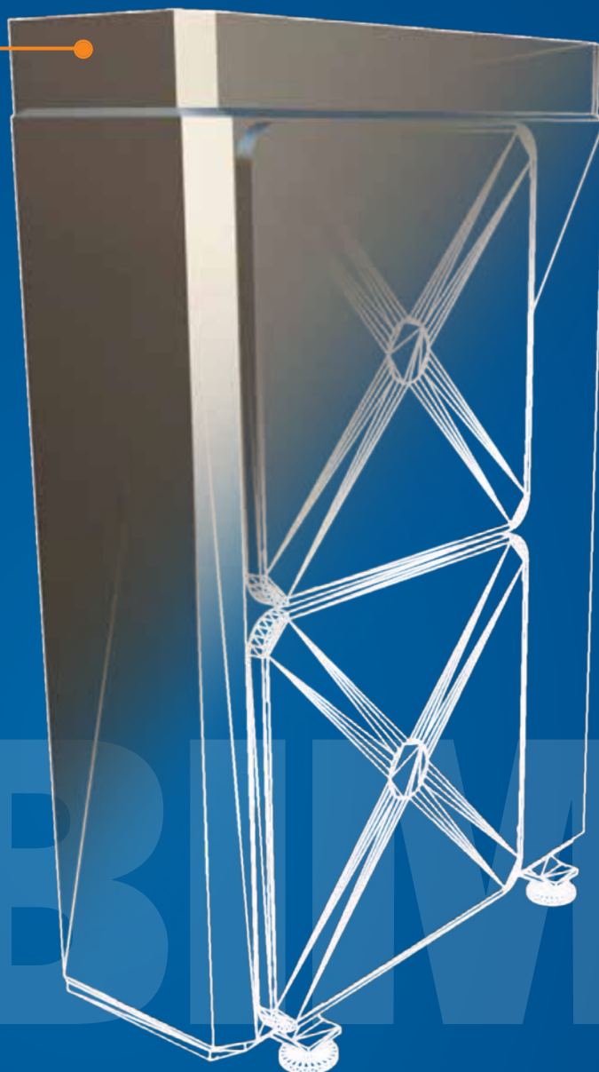
Vertex Normals
