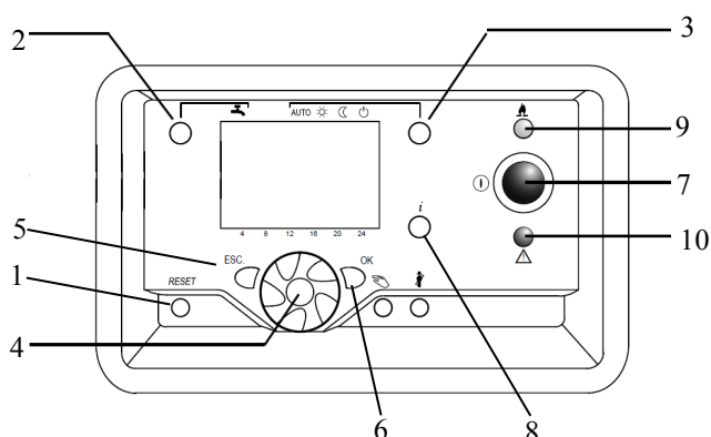
Figura 1 - Panel frontal de control de la caldera
