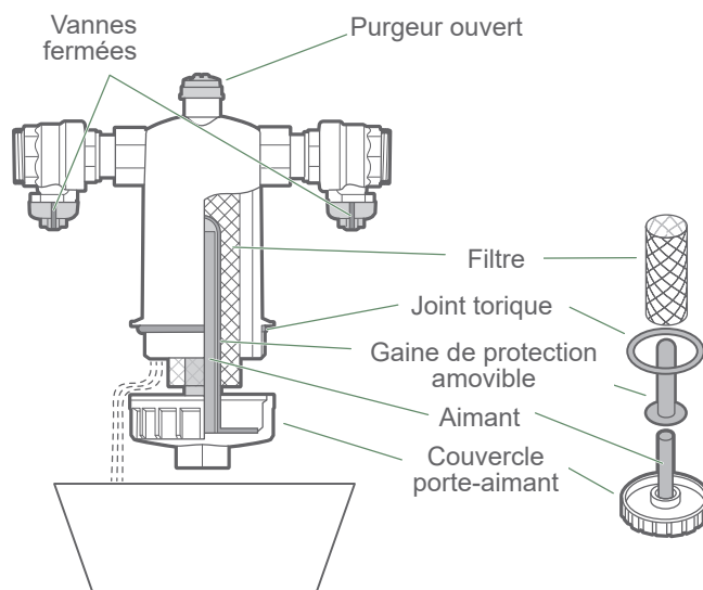
fig. 16 - Nettoyage du pot à boues
