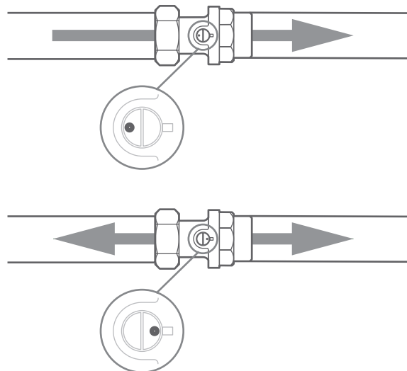
fig. 11 - Clapet antiretour
