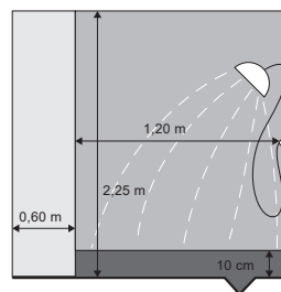
Handbrause
