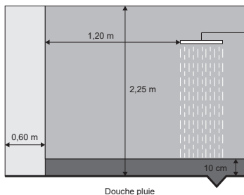
Douche pluie
