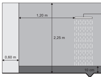
Regenbrause
