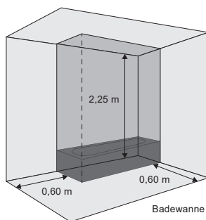
Dusche mit Wanne
