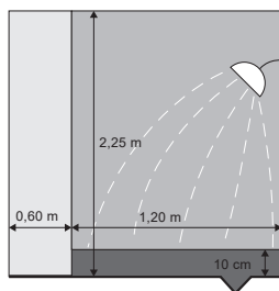
Überkopfbrause
