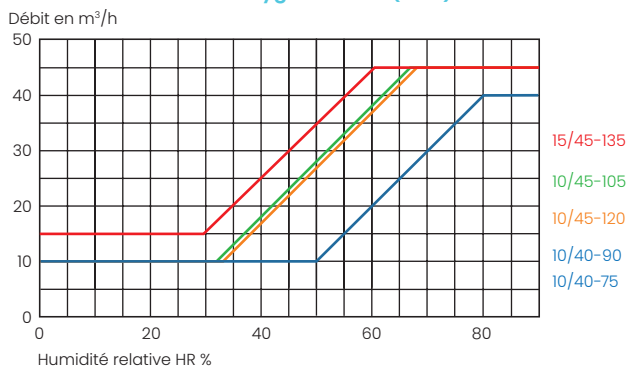
Bouche Hygro cuisine (BHC)
