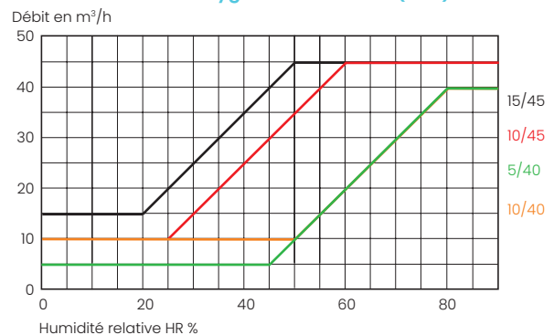
Bouche Hygro salle de bains (BHB)
