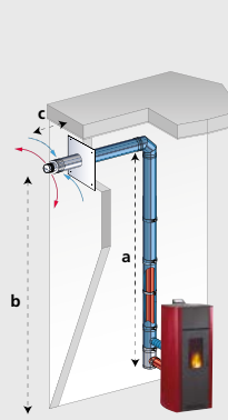
Conduit concentrique horizontal
