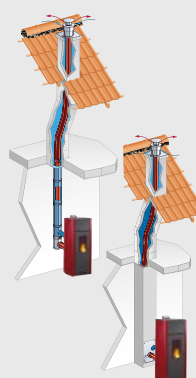
Conduit concentrique avec raccordement sur conduit existant
