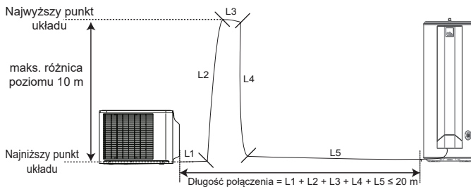
Przykładowy montaż
