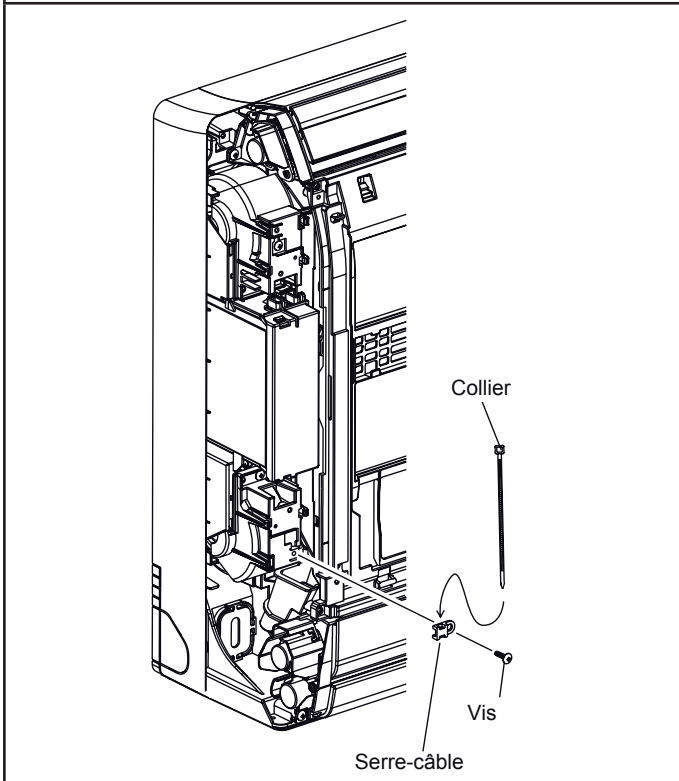
Fig. 250 - Télécommande filaire
