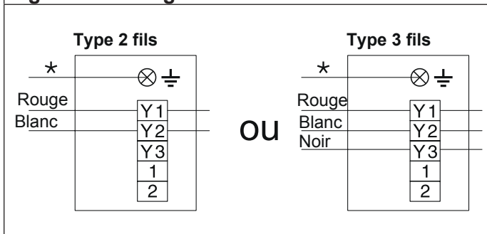
Fig. 345 : Câblage de la télécommande
