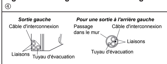
Fig. 121 - Sortie gauche ⑤ et arrière gauche ④
