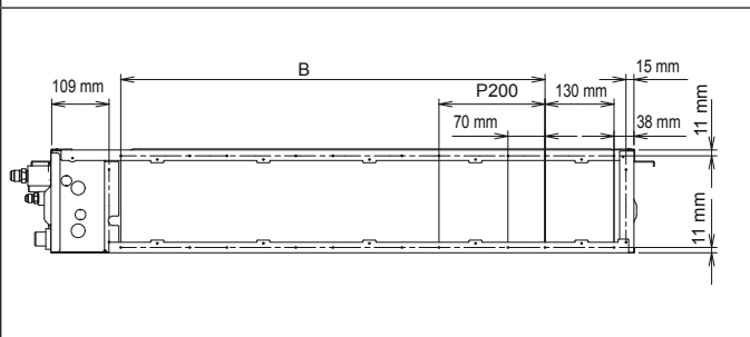
Fig. 320 - Entrée sur le côté
