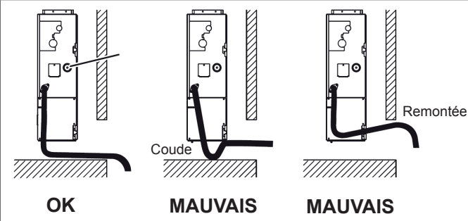
Fig. 278 - Installation au sol
