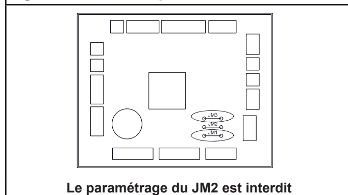
Fig. 302 - Position des ponts
