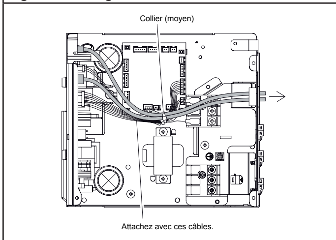
Fig. 305 - Câblage
