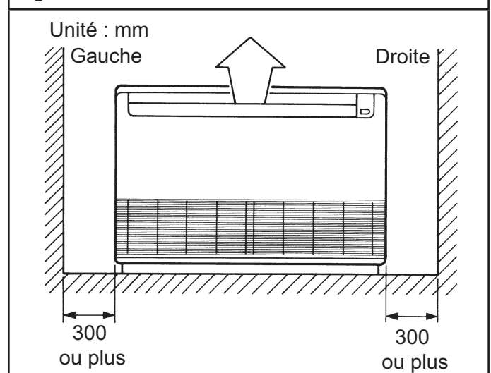
Fig. 171 - Installation en console murale
