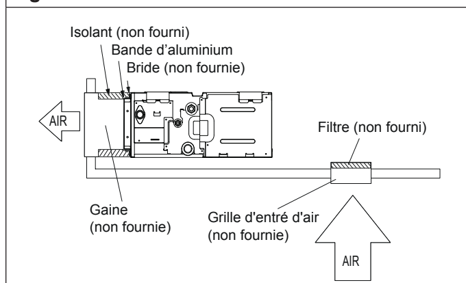
Fig. 316 - Entrée sur le côté - Sortie sur le côté
