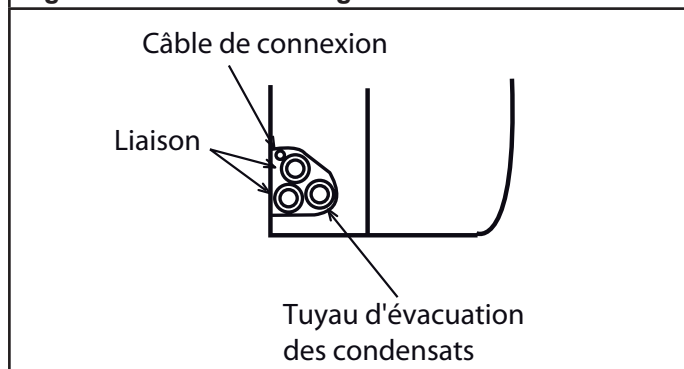
Fig. 242 - Raccordement gauche
