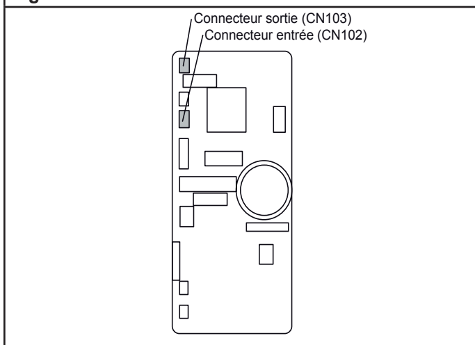
Fig. 304 - Connecteurs
