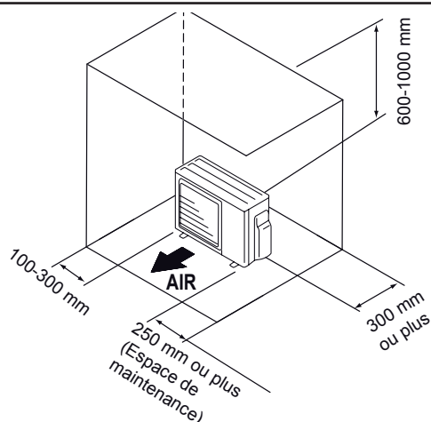
Fig. 4 - Obstacles derrière, sur un des côtés et au-dessus de l'unité
