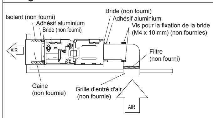
Fig. 317 - Entrée sur le côté - Sortie sur le côté avec gaine
