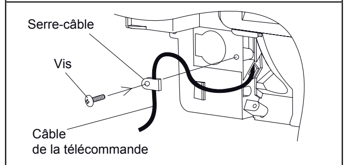
Fig. 64 - Télécommande filaire
