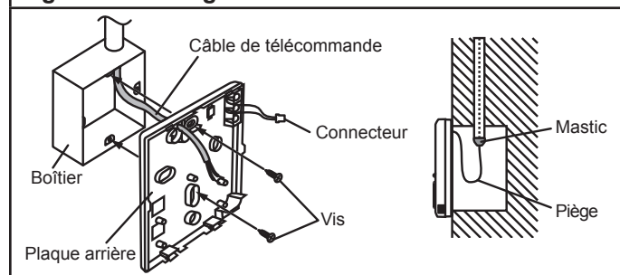
Fig. 399 - Montage avec un boîtier encastré
