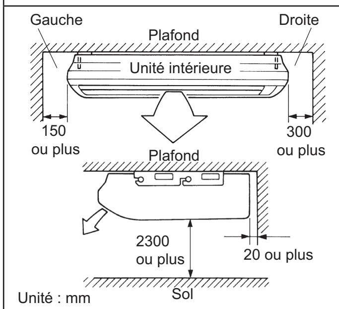
Fig. 172 - Installation en plafonnier apparent
