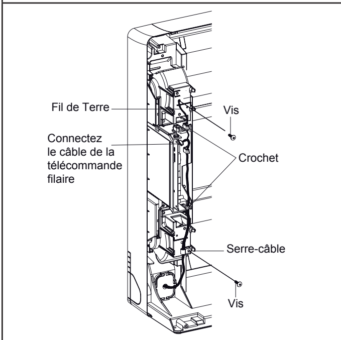
Fig. 250 - Télécommande filaire
