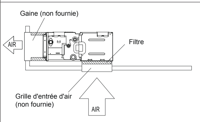
Fig. 318 - Entrée par le dessous - Sortie sur le côté
