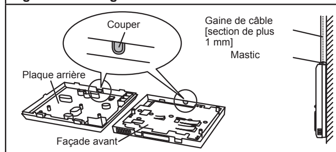
Fig. 400 - Montage direct sur un mur
