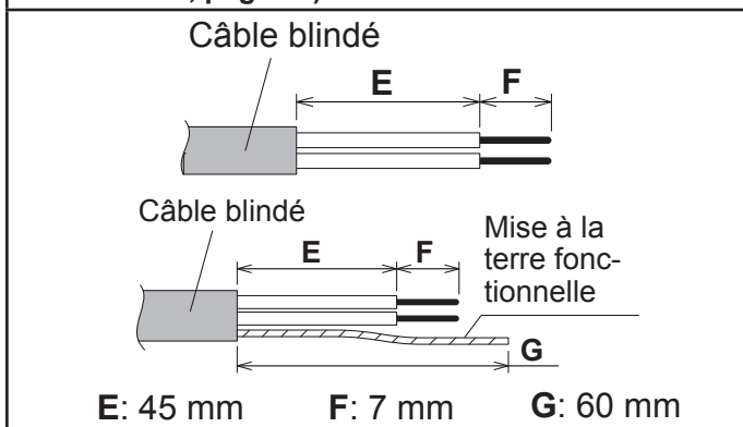
Fig. 402 - Diamètre extérieur de la gaine du câble supérieur à 5 mm - montage avec un boîtier («5.3. Installation», page 12)
