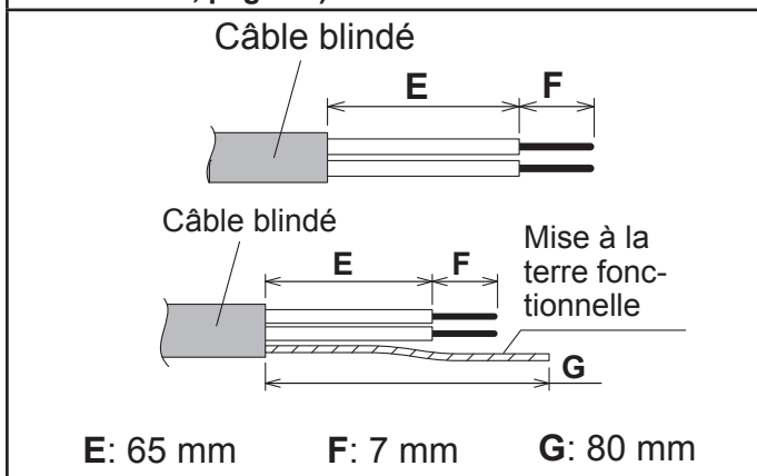
Fig. 403 - Diamètre extérieur de la gaine du câble supérieur à 5 mm - montage direct sur un mur («5.3. Installation», page 12)
