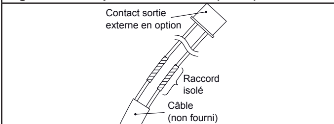
Fig. 246 - Exemple contact sortie (CN20)
