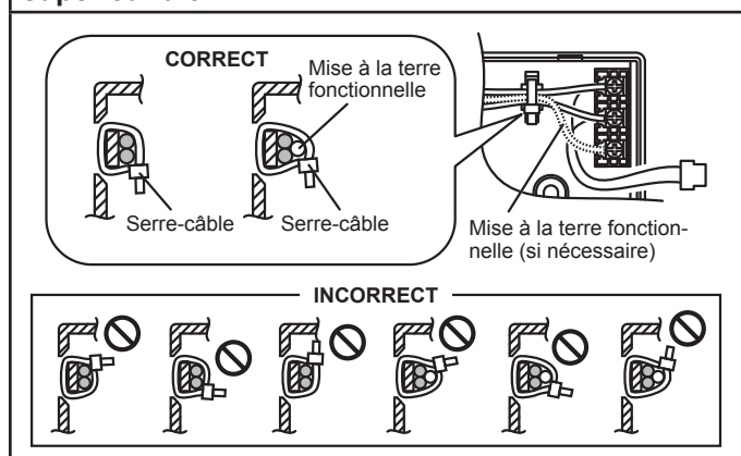
Fig. 405 - Diamètre extérieur de la gaine du câble supérieur à 5 mm
