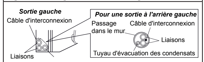
Fig. 55 - Sortie gauche ⑤ et arrière gauche ④
