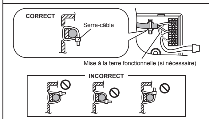
Fig. 404 - Diamètre extérieur de la gaine du câble inférieur à 5 mm
