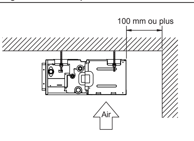
Fig. 313 Prise d'air par dessous
