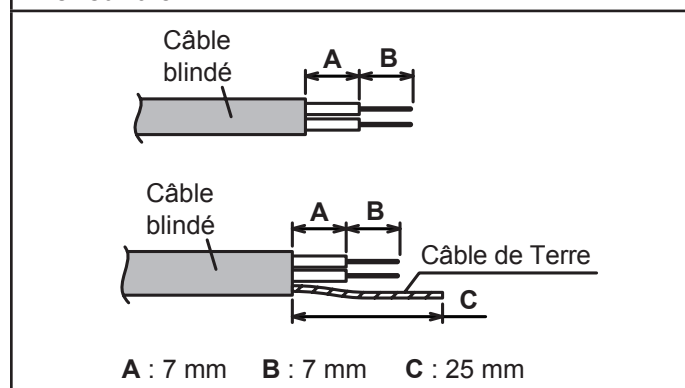
Fig. 401 - Diamètre extérieur de la gaine du câble inférieur à 5 mm
