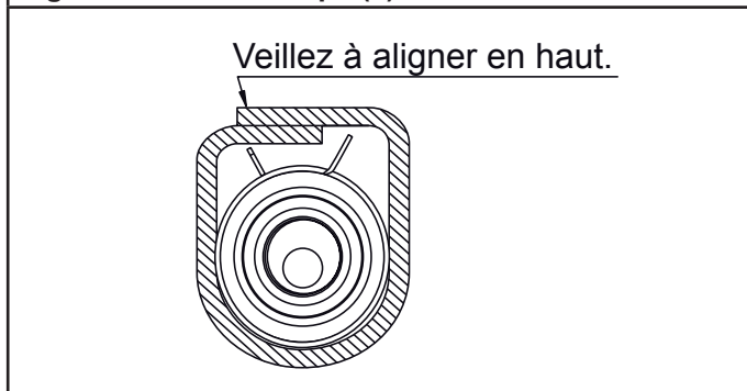
Fig. 144 - Vue en coupe (c)
