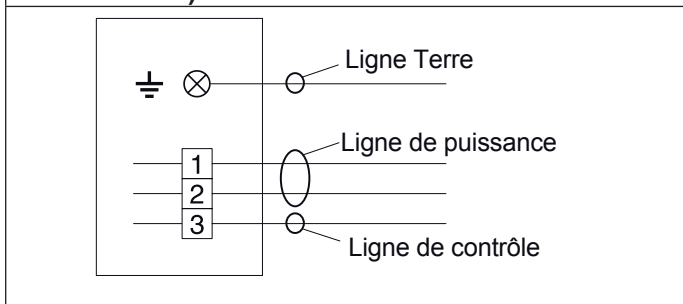
Fig. 344 : Câblage de l'interconnexion (vers l'unité extérieure)
