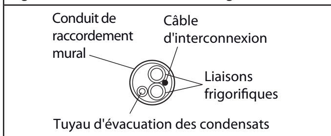
Fig. 243 - Raccordement à l'arrière gauche
