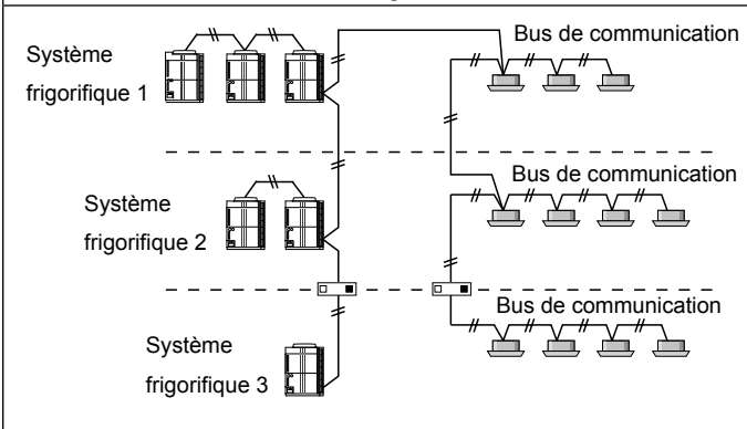
Fig. 60 - Exemple : invalider le paramétrage de l'adresse automatique
