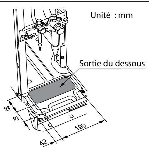
Fig. 31 - Détail de la sortie du dessous
