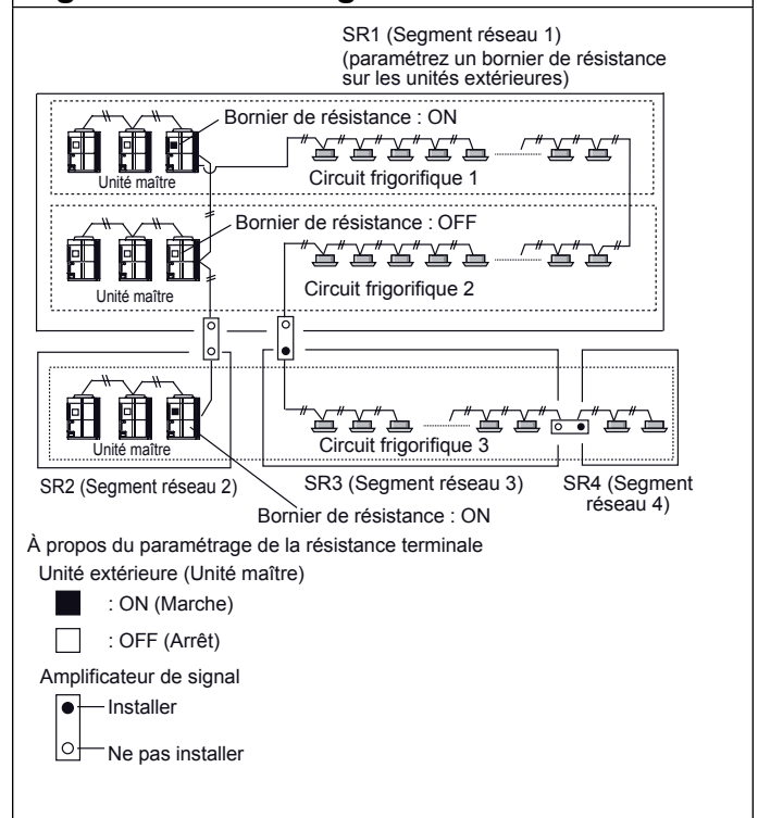
Fig. 73 - Paramétrage résistance bornier
