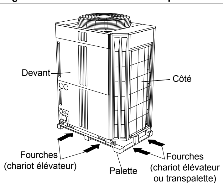
Fig. 17 - Chariot élévateur ou transpalette
