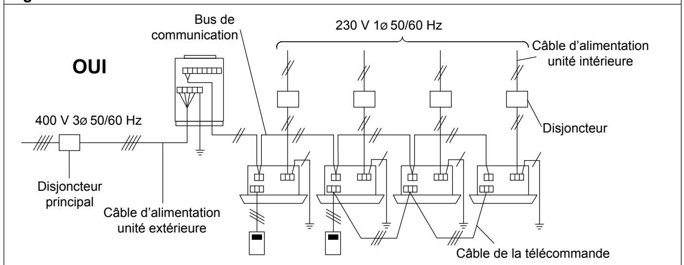
Fig. 54 - Dans le cas d'une unité extérieure connectée
