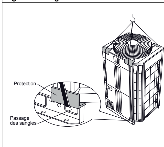
Fig. 16 - Levage
