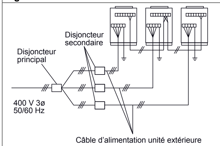
Fig. 55 - Connexion correcte
