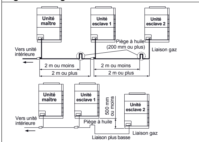
Fig. 45 - Longueur de 2 m minimum
