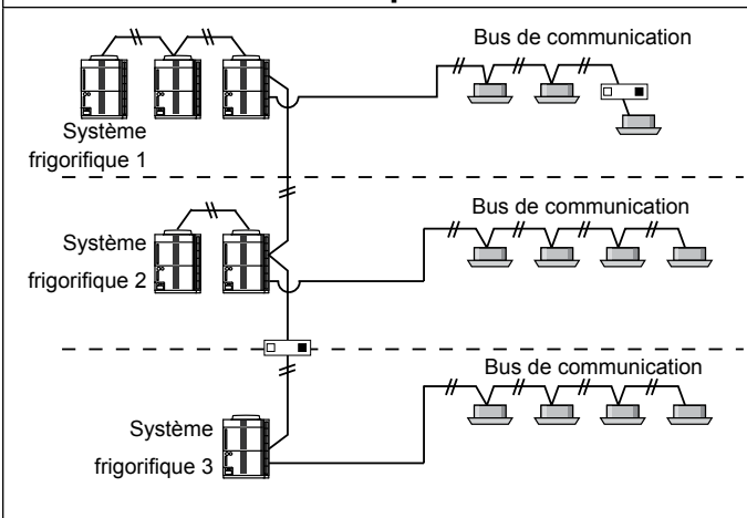
Fig. 61 - Exemple : valider le paramétrage de l'adresse automatique
