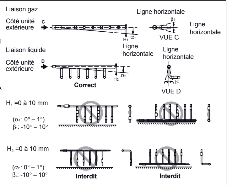
Fig. 28 - Répartiteurs
