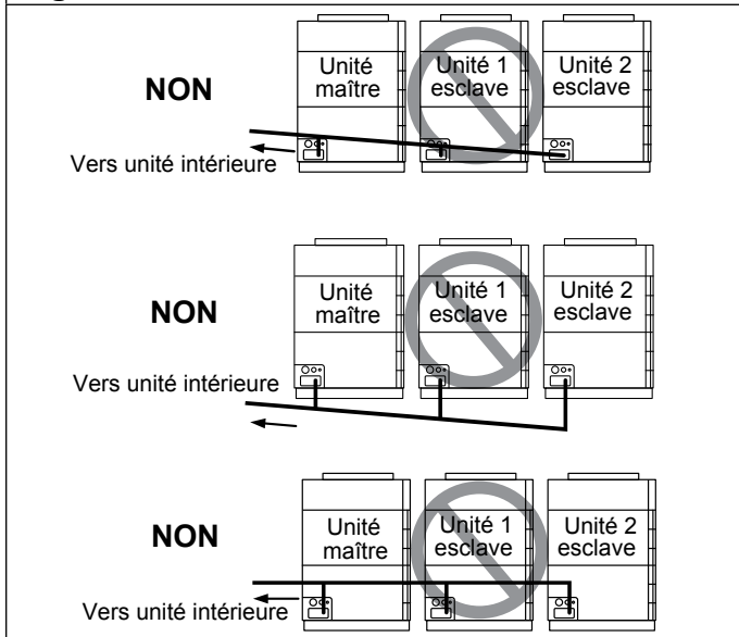
Fig. 43 - Mauvaises installations
