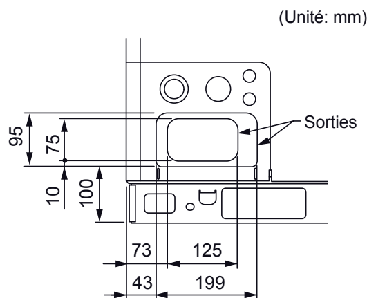
Fig. 32 - Détail de la sortie de devant
