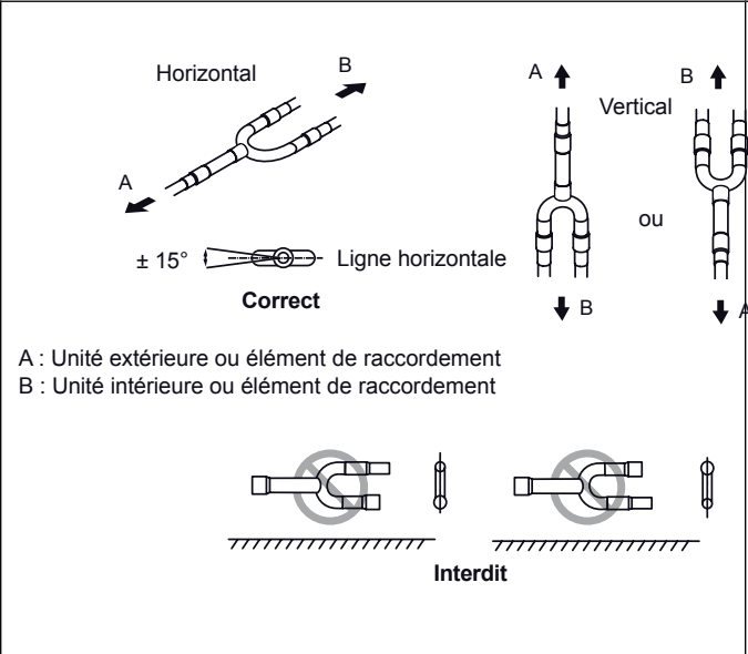
Fig. 27 - Séparateurs
