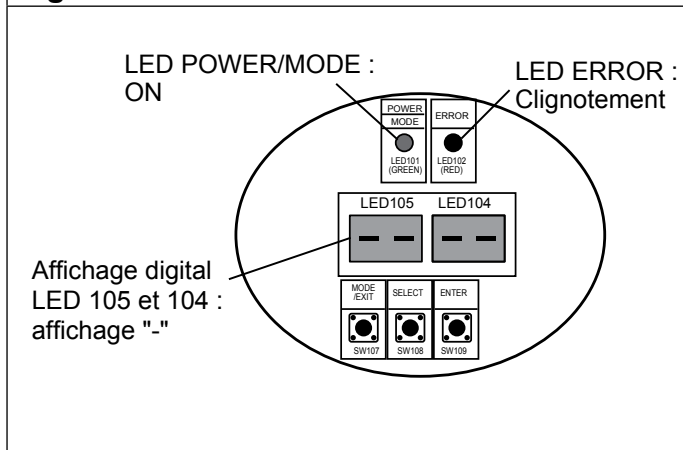
Fig. 75 - Fonctionnement anormal
