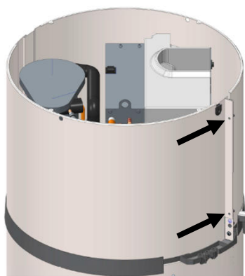
Aflojar los 2 tornillos de tapa delantera
