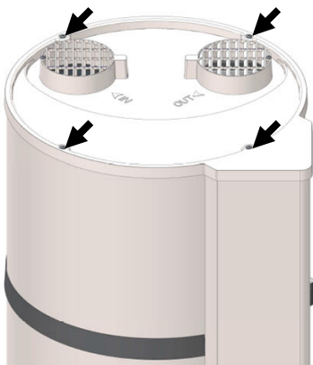
Aflojar los 4 tornillos de tapa
