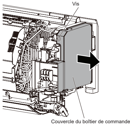
Couvercle du boîtier de commande
