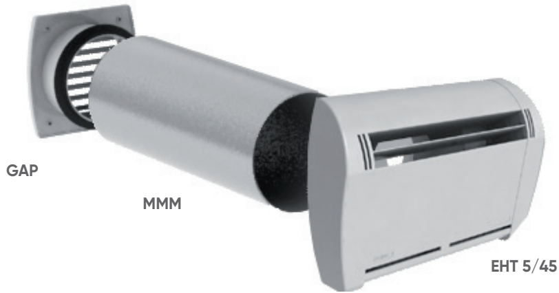
Exemple de montage dans un mur épaisseur 300 mm à 125 mm.
