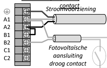
Schema inqana droog
