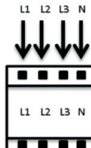
Raccordement sur interrupteur de proximité (P SW 4000/5000 - 3 x 400 V + N)
