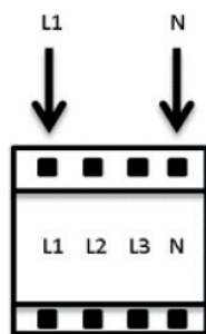
Raccordement sur interrupteur de proximité (P SW 500 - 1 x 230 V)
