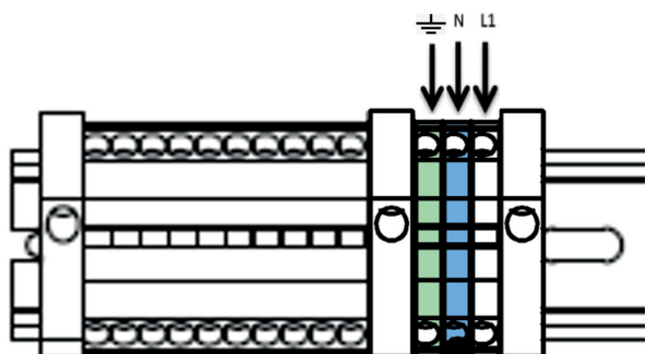
Raccordement sur bornier (P SW 1000/2000 - 1 x 230 V)
