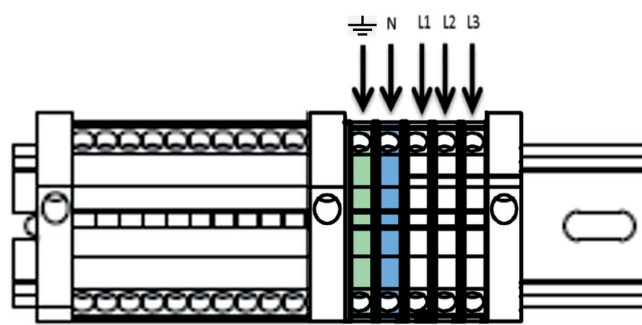
Raccordement sur bornier (P SW 2500/3000 - 3 x 400 V + N)
