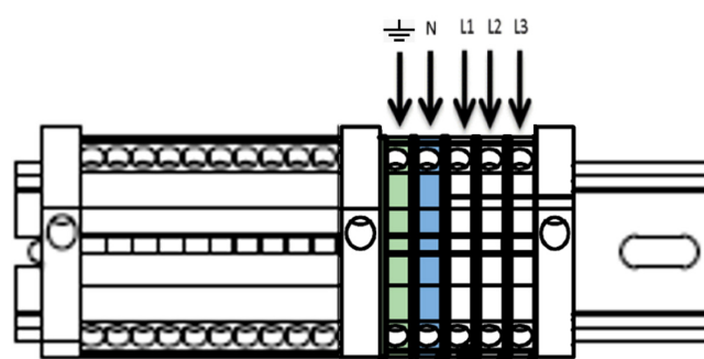
Raccordement sur bornier (P SW 2500/3000 - 3 x 400 V + N)
