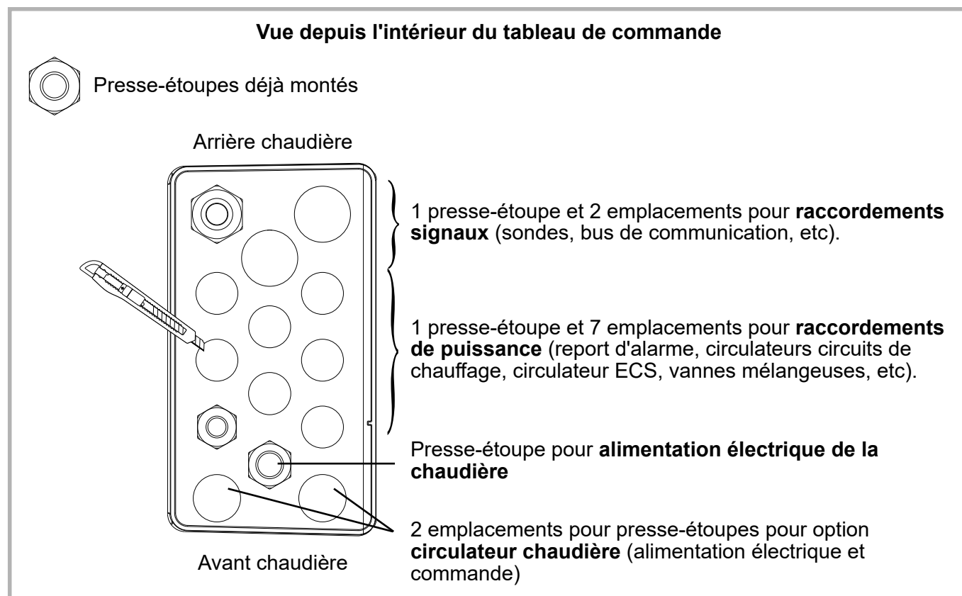
figure 23 - Presse-étoupes
