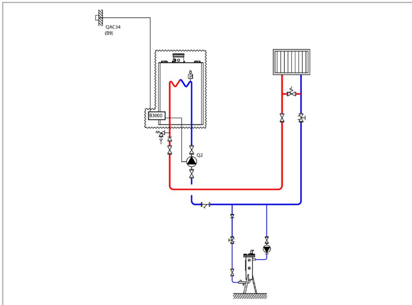
figure 32 - Schéma VF20
