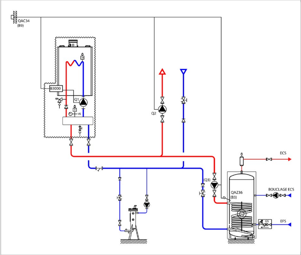
figure 29 - Schéma VF2
