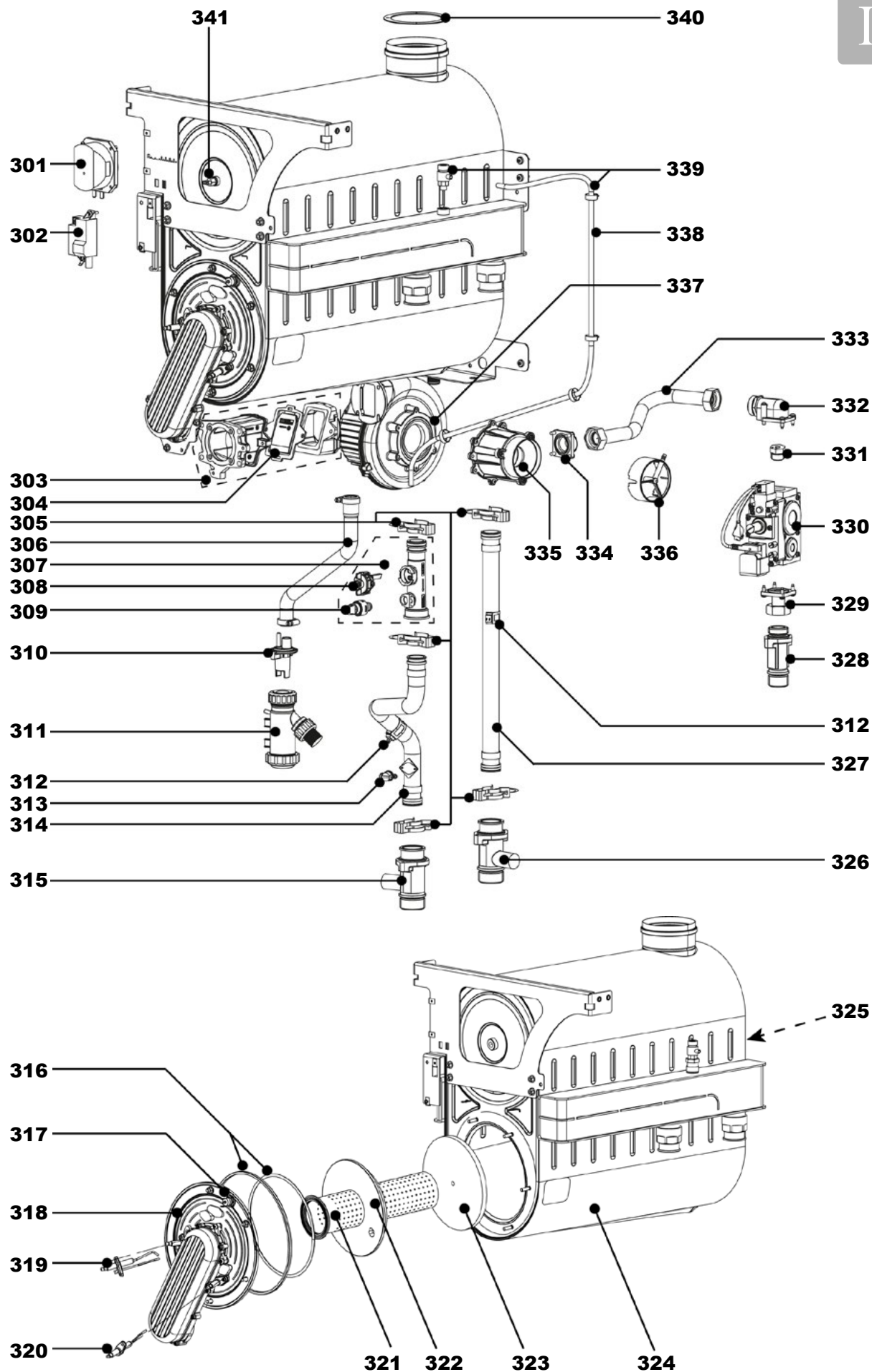
figure 42 - Corps et brûleur modèles 70 à 120
