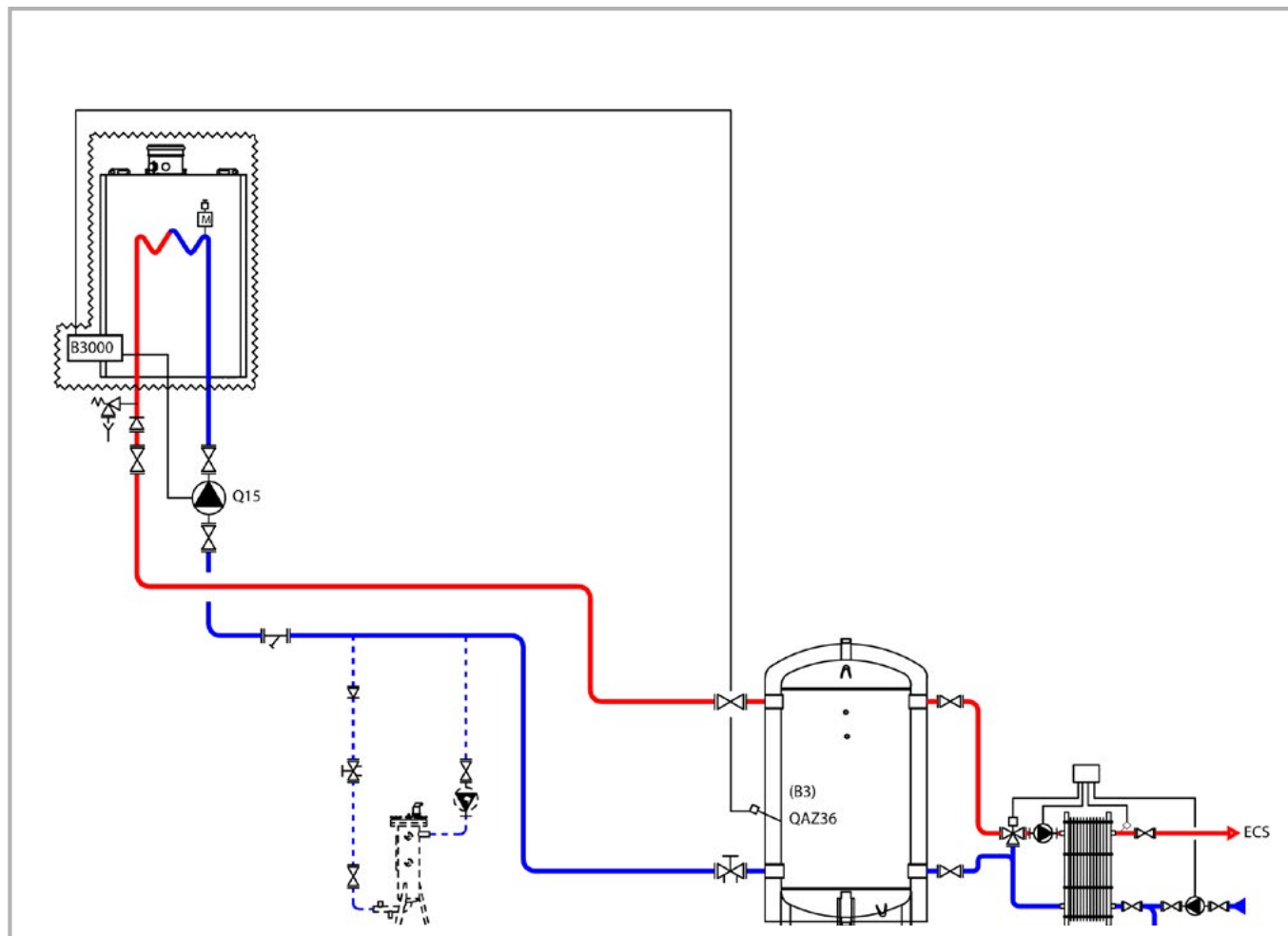
figure 35 - Schéma VF23
