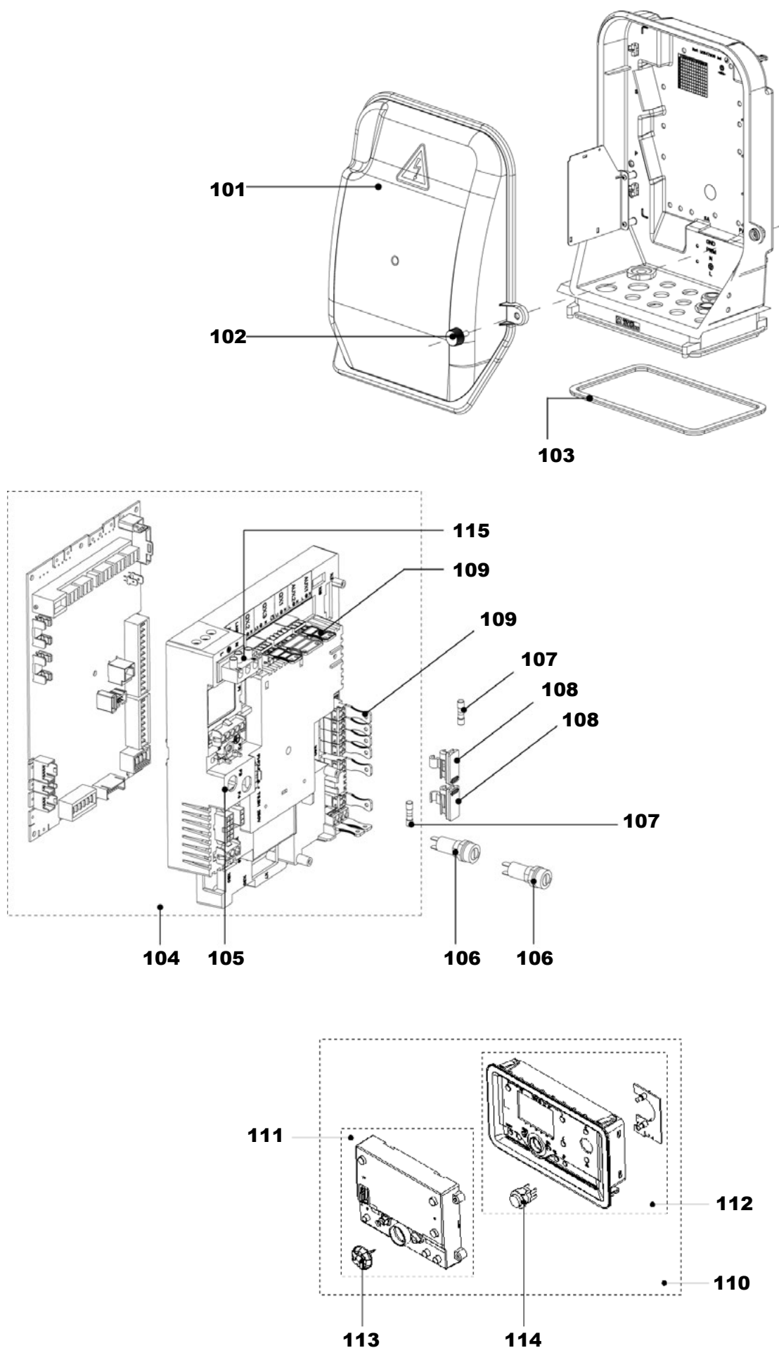
figure 40 - Tableau de commande
