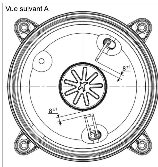
figure 26 - Position électrodes brûleur
