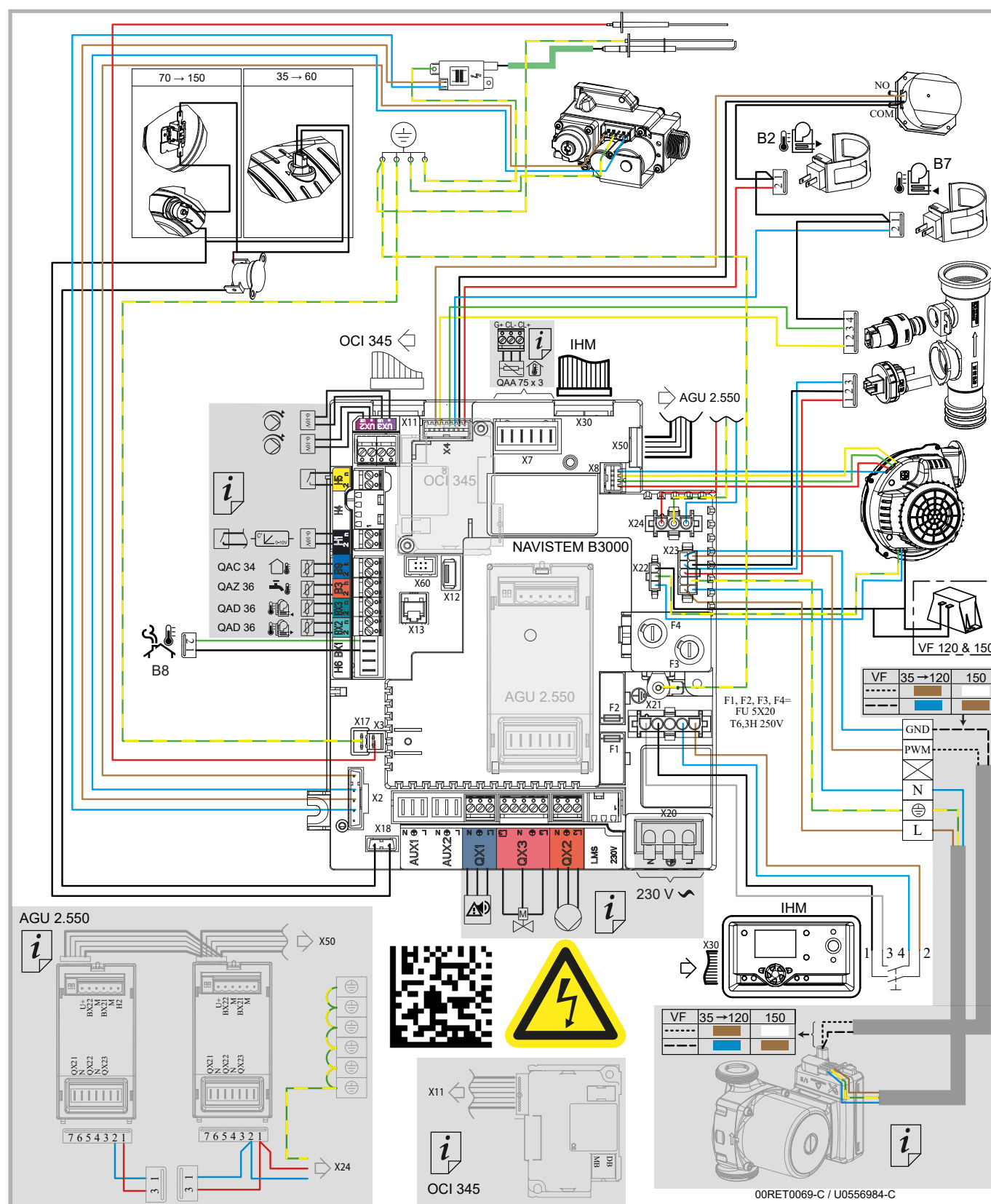
figure 23 - Schéma électrique
