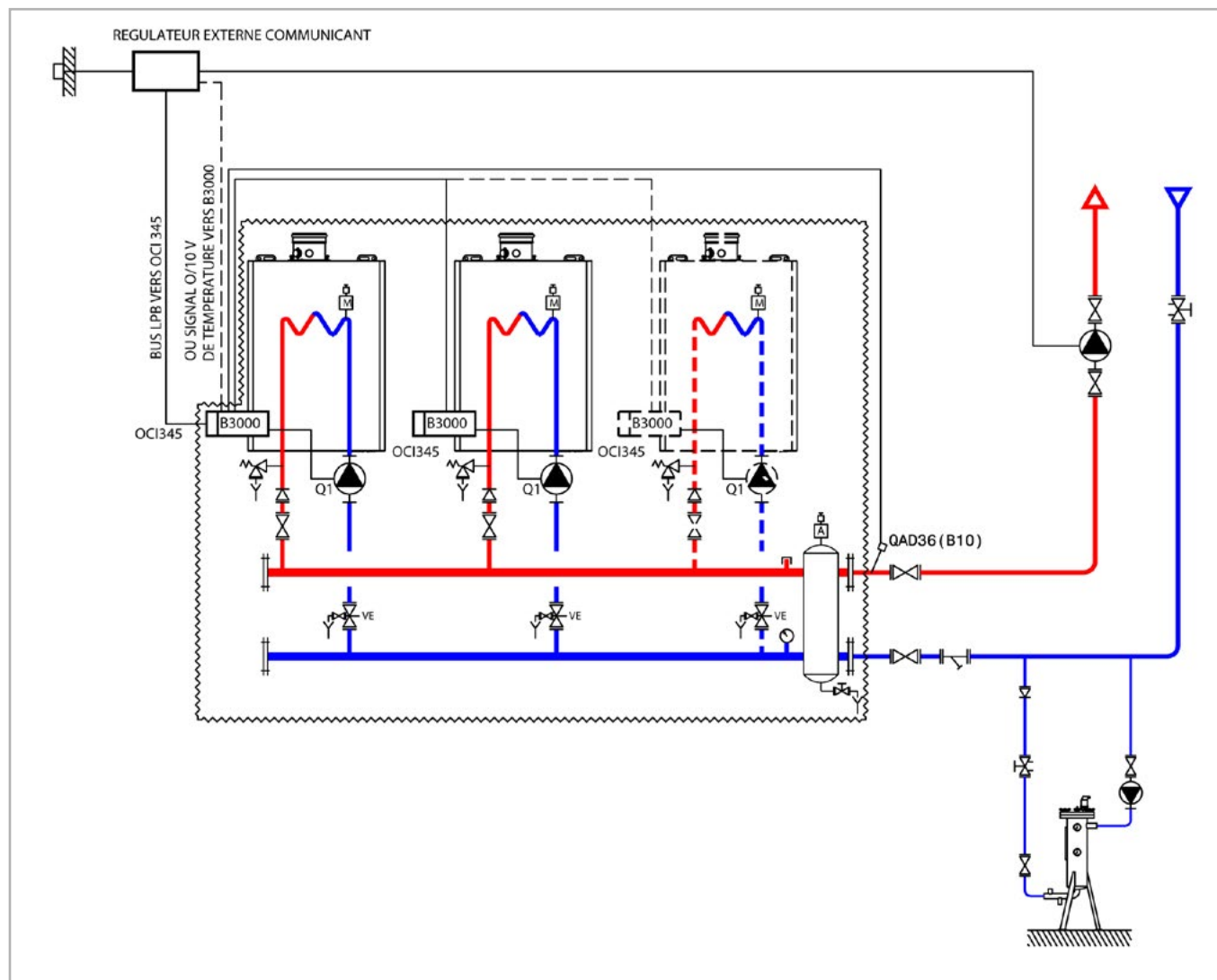
figure 37 - Schéma VF10
