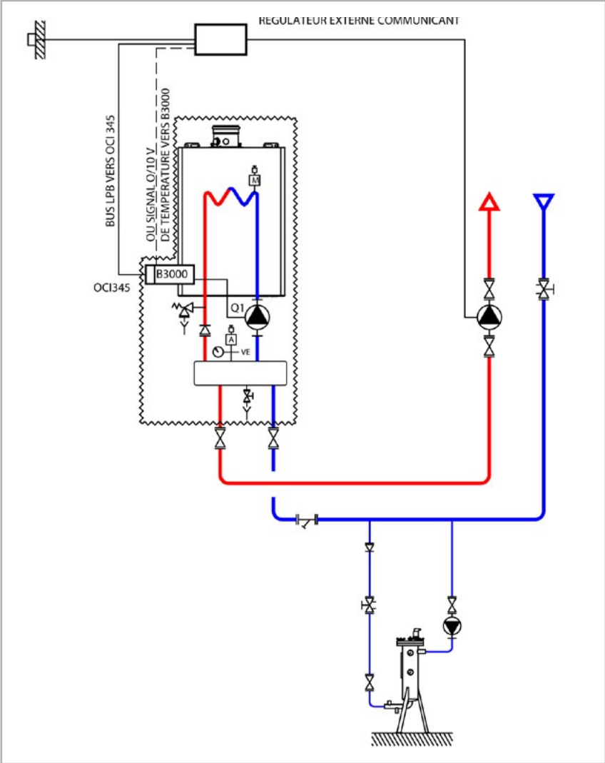
figure 28 - Schéma VF1
