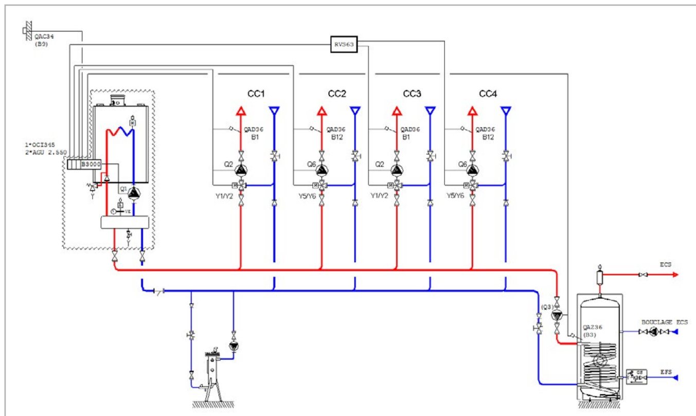
figure 31 - Schéma VF4
