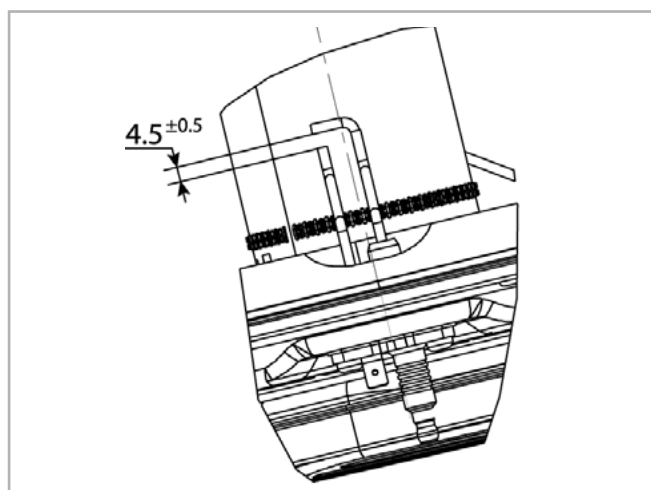
figure 27 - Géométrie électrode
