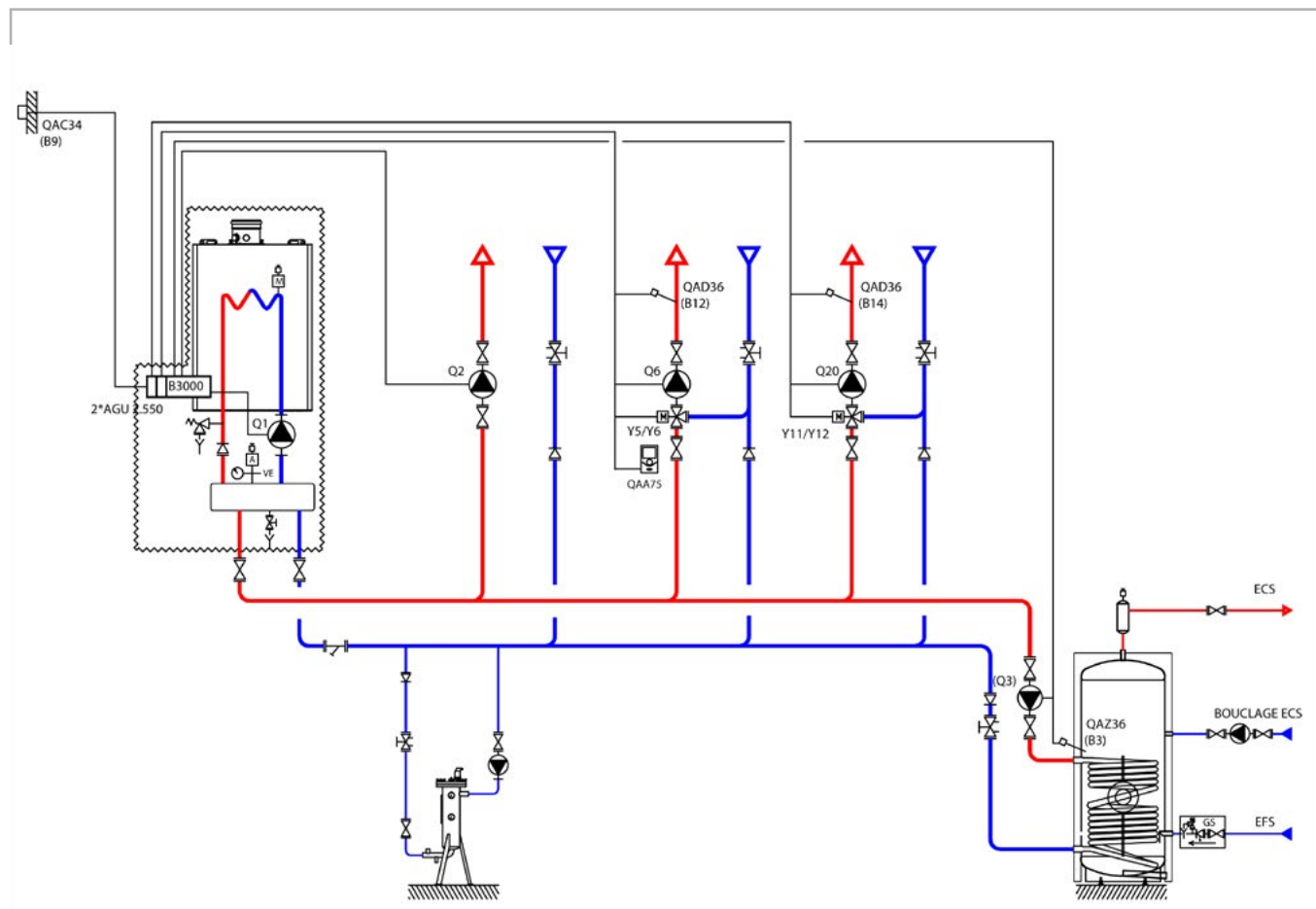
figure 30 - Schéma VF3
