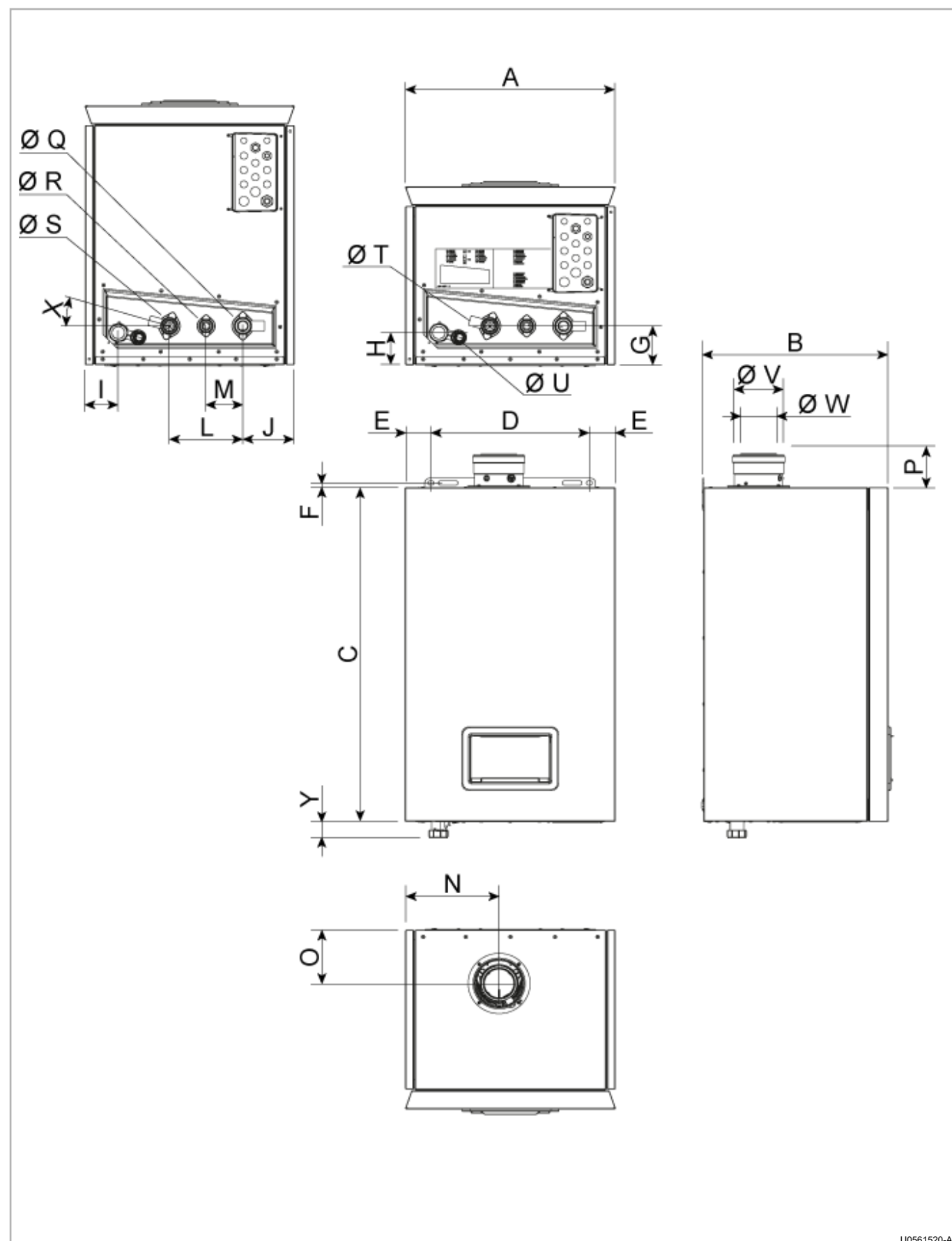
figure 1 - Caractéristiques dimensionnelles
