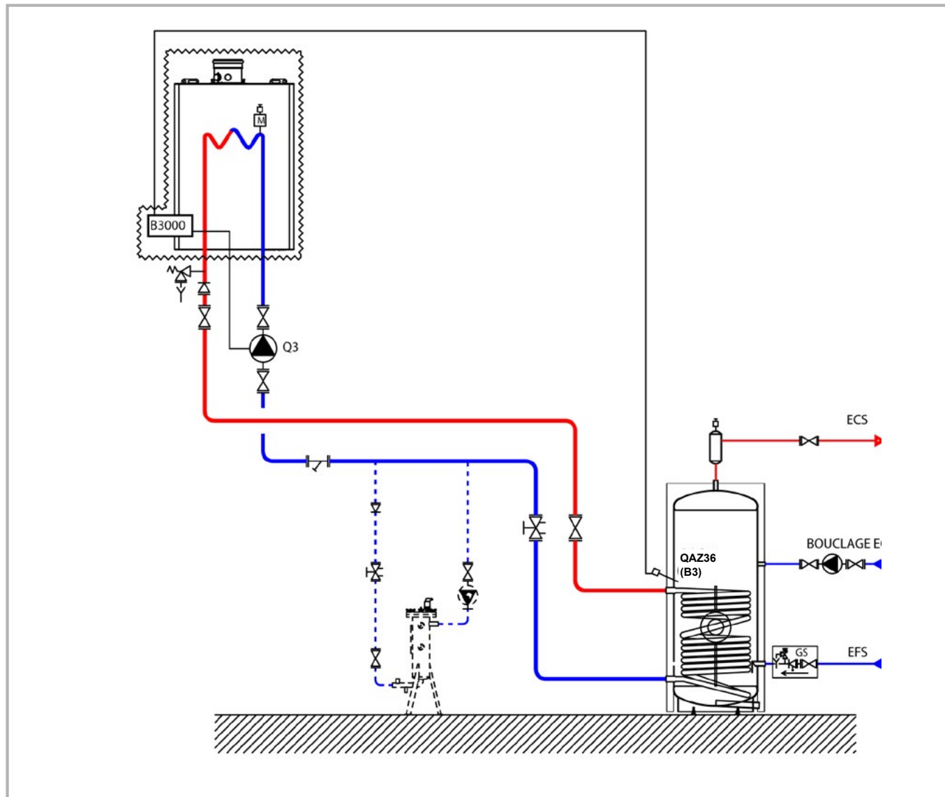
figure 36 - Schéma VF24
