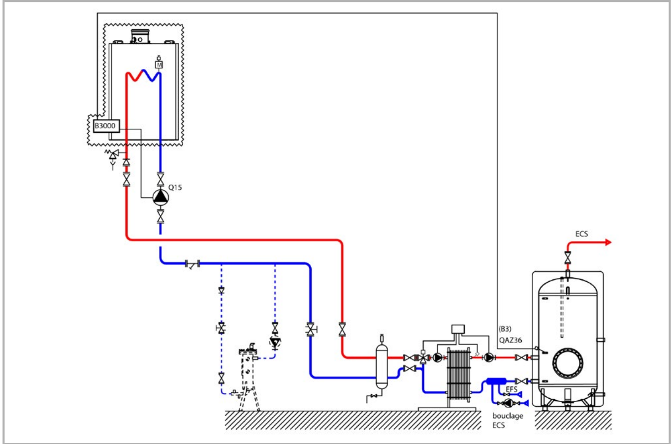
figure 34 - Schéma VF22
