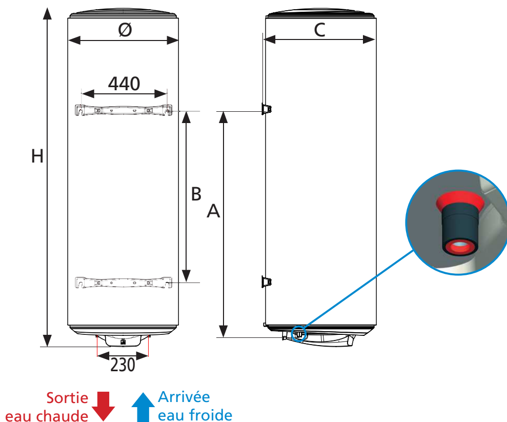
Représentation schématique
