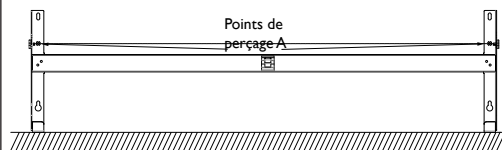
Modèle Plinthe
